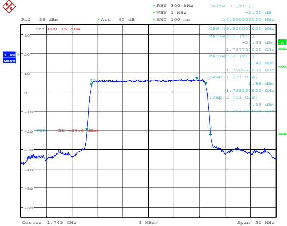
QPSK
