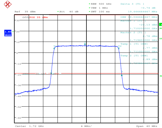
16-QAM
