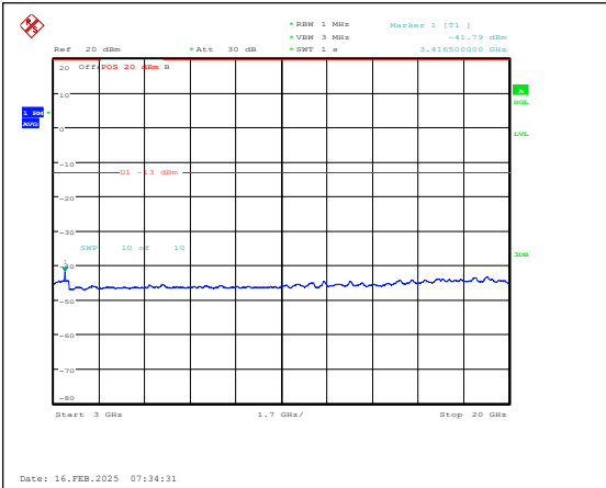
Band4-20MHz-QPSK-20050-1RB#0-3000~20000 -PASS
