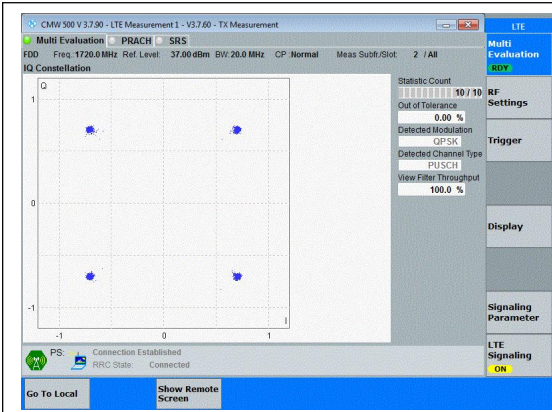
Band4-20MHz-QPSK-20050-100RB#0-PASS
