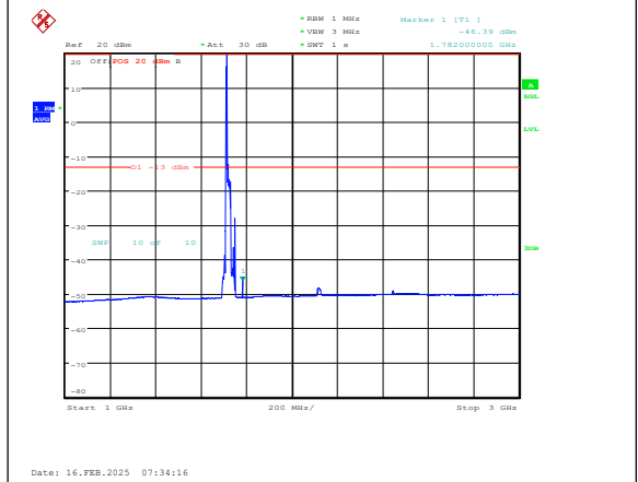
Band4-20MHz-QPSK-20050-1RB#0-1000~3000-P ASS
