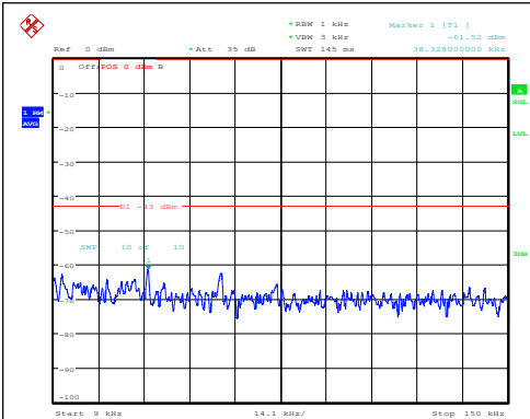
Band4-20MHz-QPSK-20175-1RB#0-0.009~0.15-PASS
