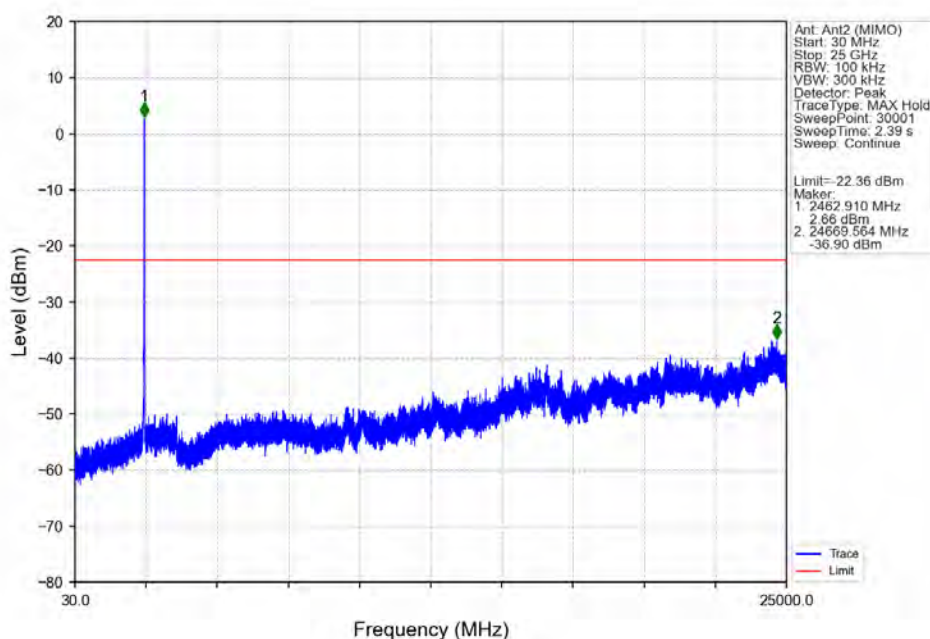
802.11ac(VHT20) HCH 2462MHz Ant2 (MIMO) NTN
