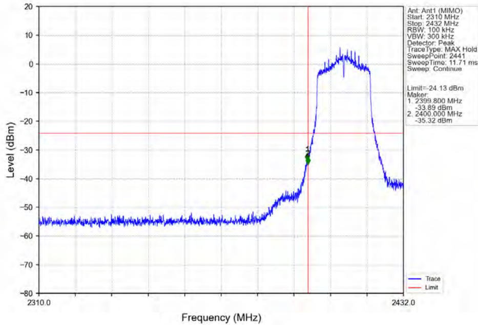
802.11ac(VHT20) LCH 2412MHz Ant1 (MIMO) NTN
