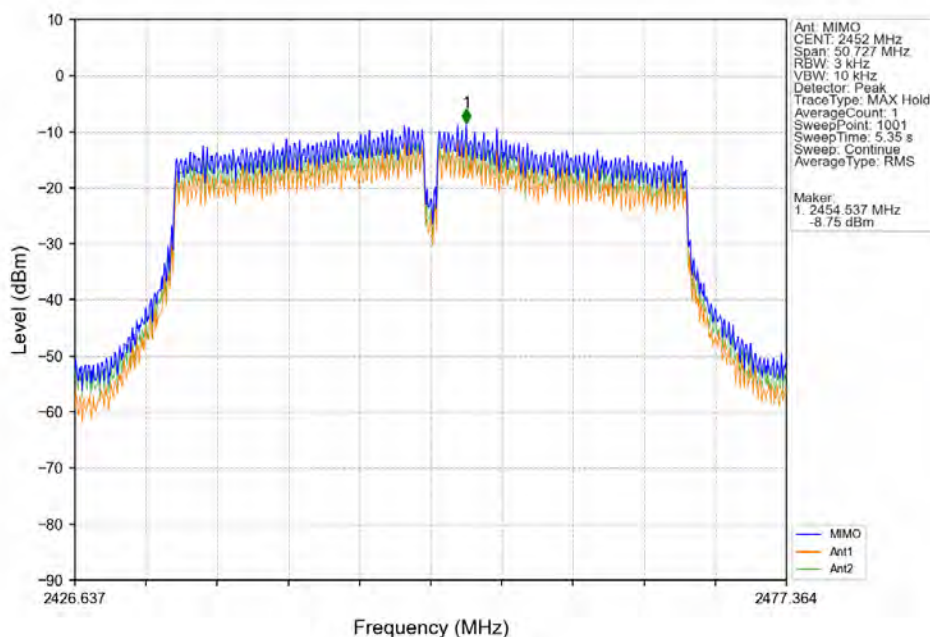
802.11ac(VHT40) HCH 2452MHz MIMO NTN
