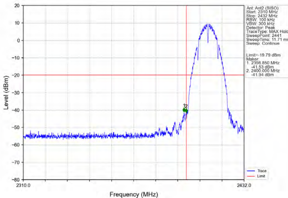
802.11b_LCH_2412MHz_Ant2 (SISO)_NTNV
