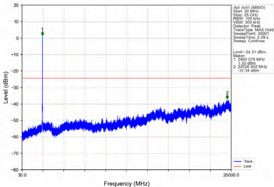
802.11ax(HEW20) HCH 2462MHz SU / Ant1 (MIMO) NTN
