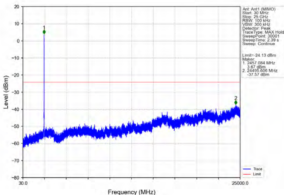
802.11ac(VHT20) HCH 2462MHz Ant1 (MIMO) NTN
