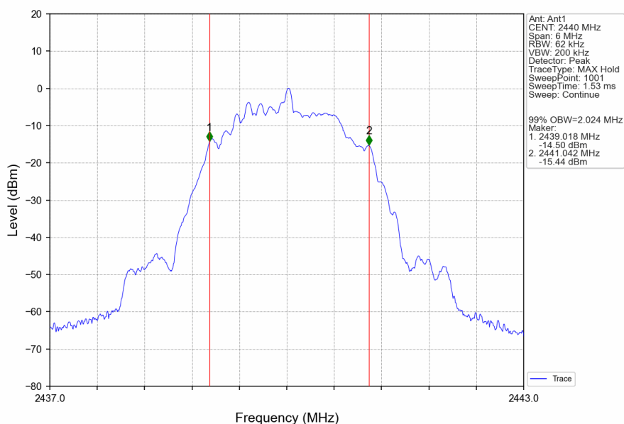
2M_MCH_2440MHz_Ant1_NTNV
