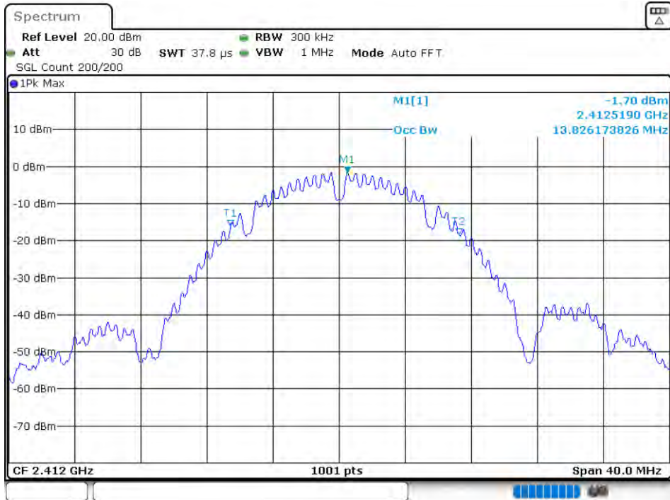
OBW NVHT 802.11b 2412MHz Ant1
