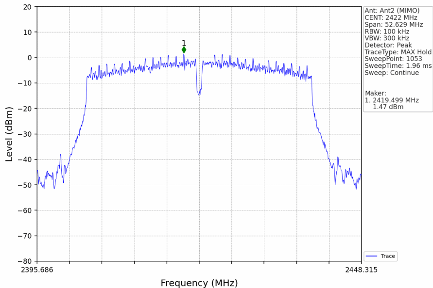
802.11n(HT40)_LCH_2422MHz_Ant2 (MIMO)_NTNV
