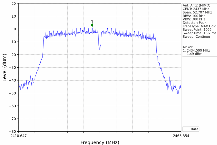
802.11n(HT40)_MCH_2437MHz_Ant2 (MIMO)_NTNV
