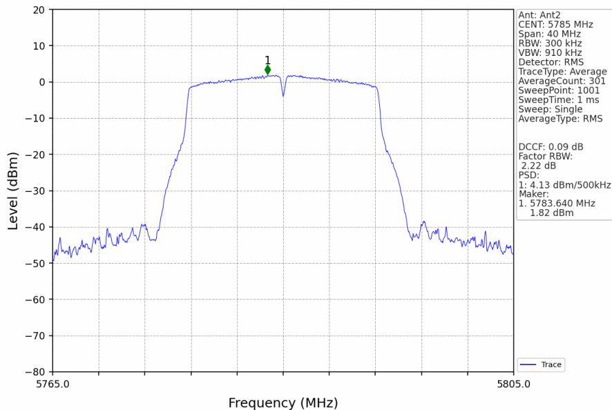
802.11a_MCH_5785MHz_Ant2_NTNV
