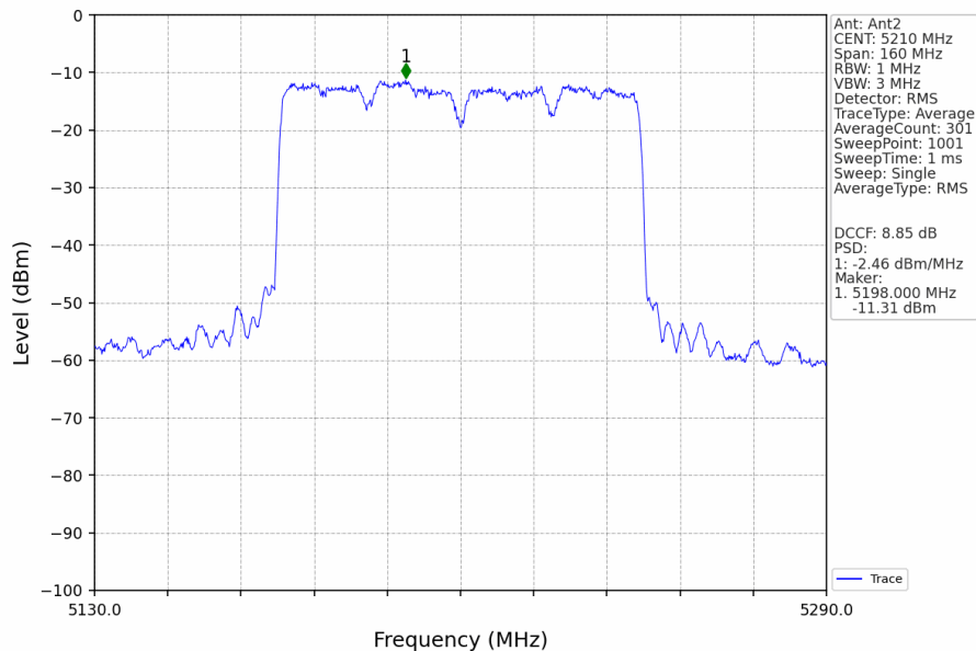
802.11ax(HEW80)_MCH_5210MHz_RU996_Left_Ant2_NTNV
