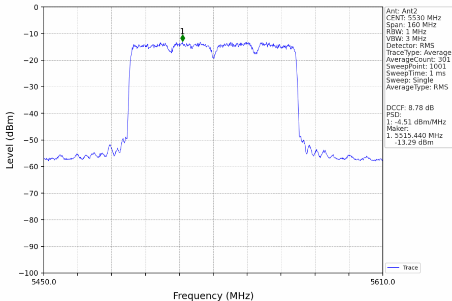
802.11ax(HEW80)_LCH_5530MHz_RU996_Left_Ant2_NTNV
