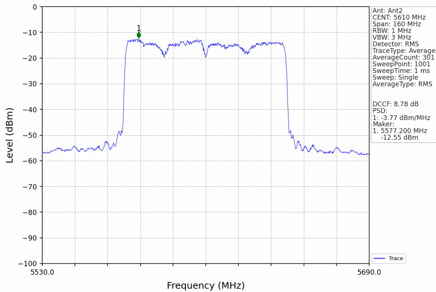
802.11ax(HEW80)_HCH_5610MHz_RU996_Left_MIMO_NTNV
