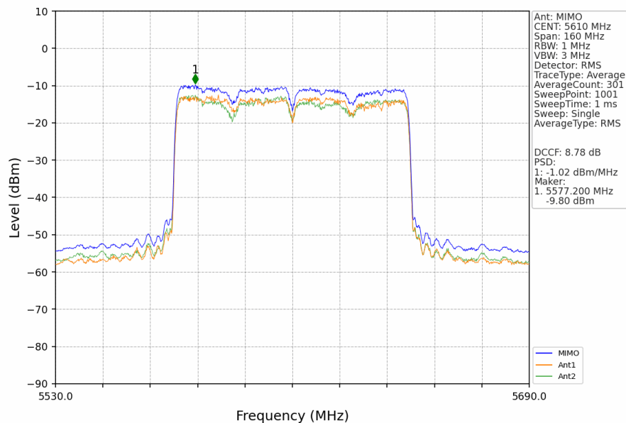
802.11ax(HEW80)_HCH_5610MHz_RU996_Left_MIMO_NTNV
