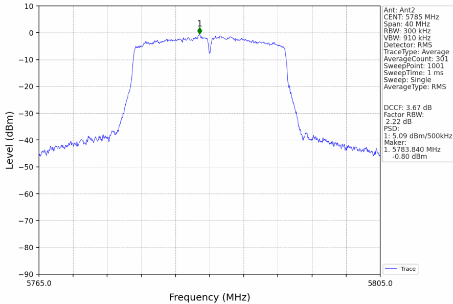
802.11n(HT20)_MCH_5785MHz_MIMO_NTNV
