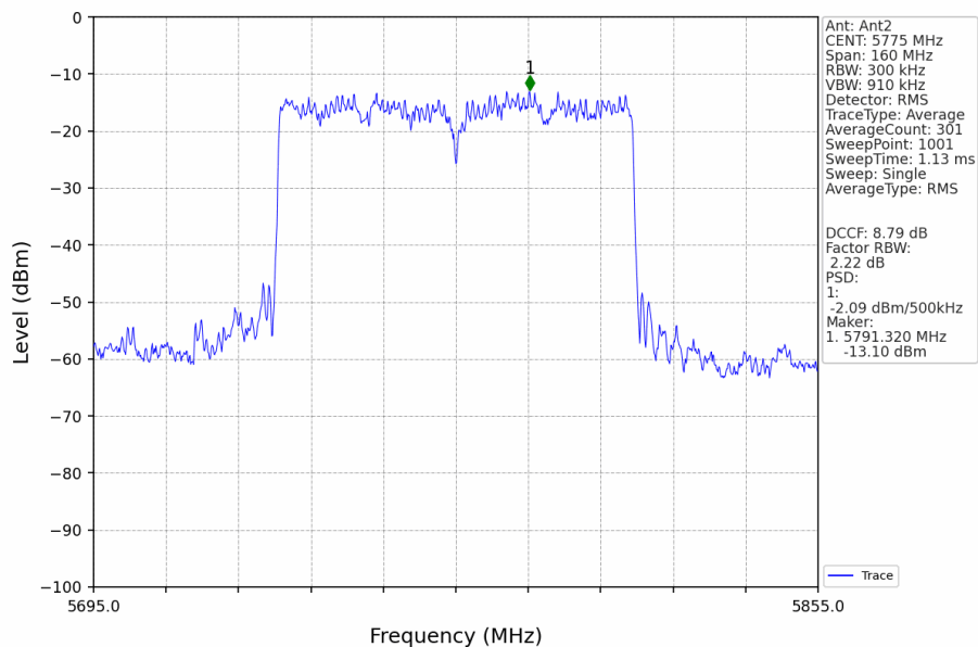
802.11ax(HEW80)_MCH_5775MHz_RU996_Left_Ant2_NTNV
