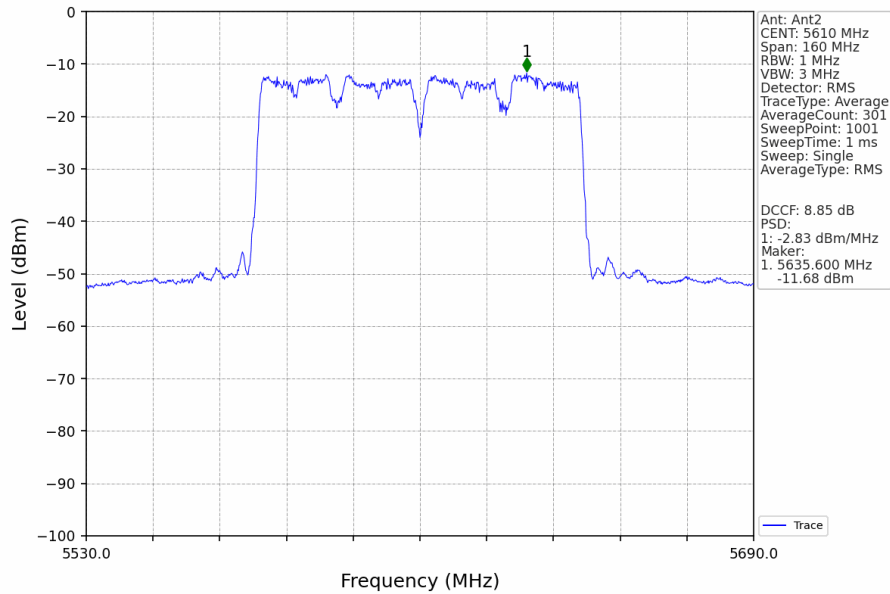
802.11ac(VHT80)_HCH_5610MHz_MIMO_NTNV
