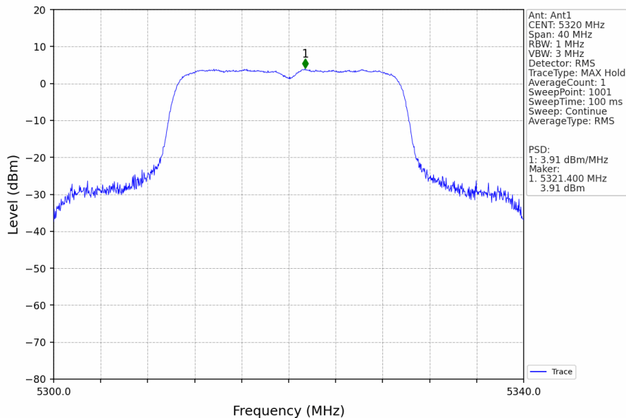
802.11ax(HEW20)_HCH_5320MHz_RU242_Left_Ant1_NTNV
