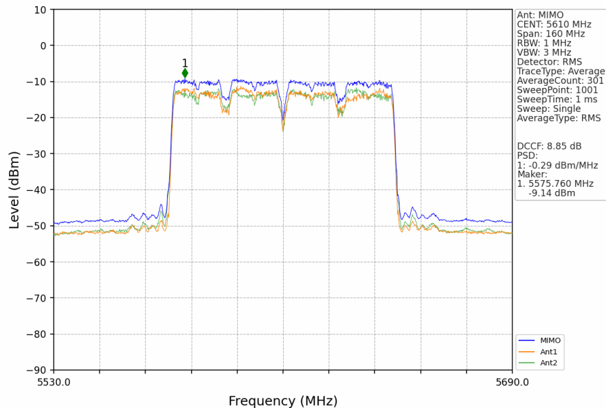
802.11ac(VHT80)_HCH_5610MHz_MIMO_NTNV
