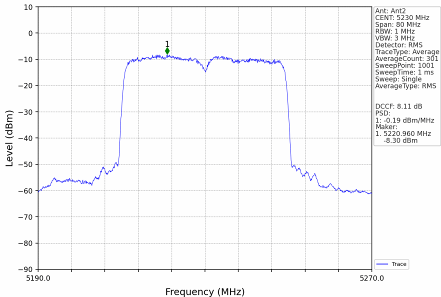
802.11ax(HEW40)_HCH_5230MHz_RU484_Left_Ant2_NTNV
