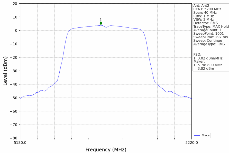
802.11n(HT20)_MCH_5200MHz_MIMO_NTNV
