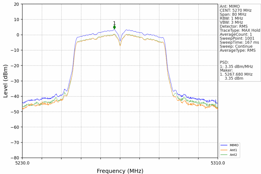
802.11n(HT40)_LCH_5270MHz_MIMO_NTNV
