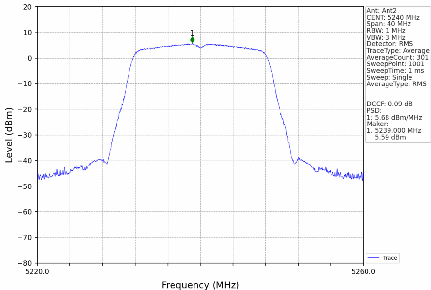
802.11a_HCH_5240MHz_Ant2_NTNV
