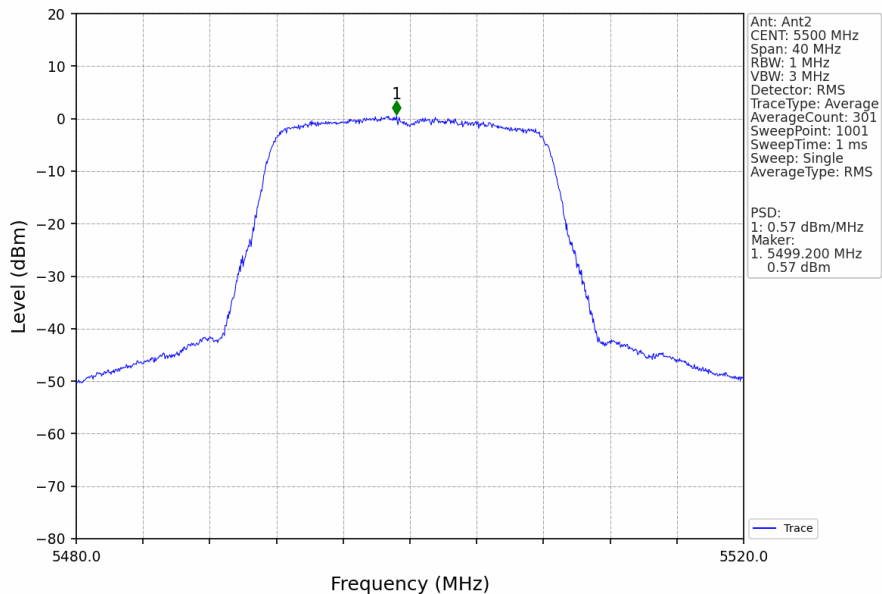
802.11a_LCH_5500MHz_Ant2_NTNV
