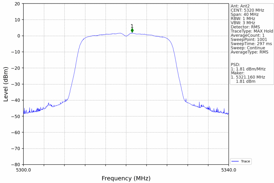
802.11n(HT20)_HCH_5320MHz_MIMO_NTNV
