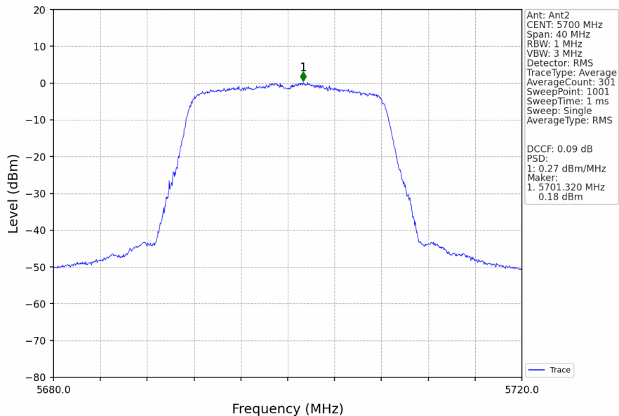
802.11a_HCH_5700MHz_Ant2_NTNV
