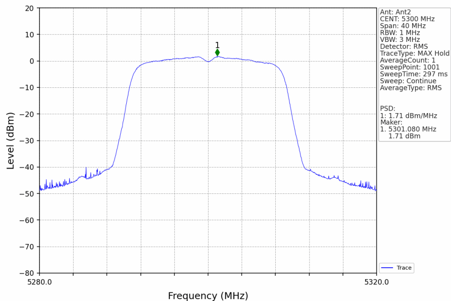
802.11n(HT20)_MCH_5300MHz_Ant2_NTNV
