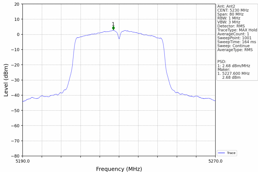
802.11n(HT40)_HCH_5230MHz_Ant2_NTNV
