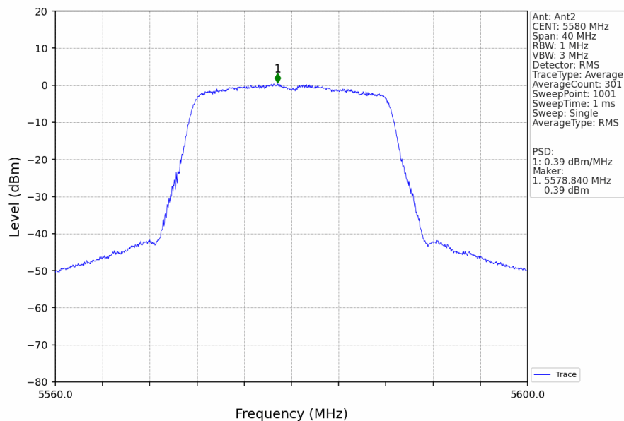
802.11a_MCH_5580MHz_Ant2_NTNV
