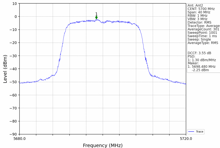
802.11n(HT20)_HCH_5700MHz_Ant2_NTNV
