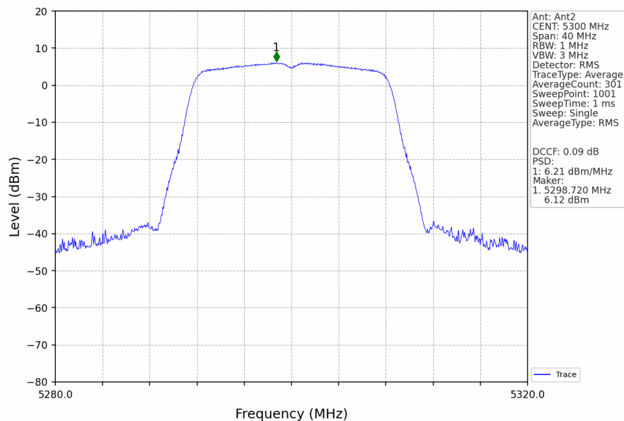
802.11a_MCH_5300MHz_Ant2_NTNV
