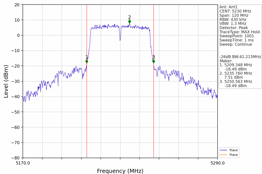
802.11ac(VHT40)_HCH_5230MHz_Ant1_NTNV
