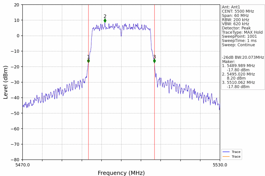
802.11ax(HEW20)_LCH_5500MHz_RU242_Left_Ant1_NTNV
