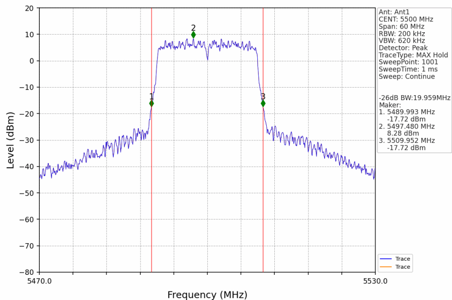
802.11ac(VHT20)_LCH_5500MHz_Ant1_NTNV
