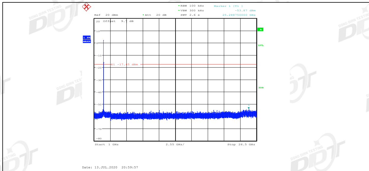
11B_Ant2_2462_0~Reference
