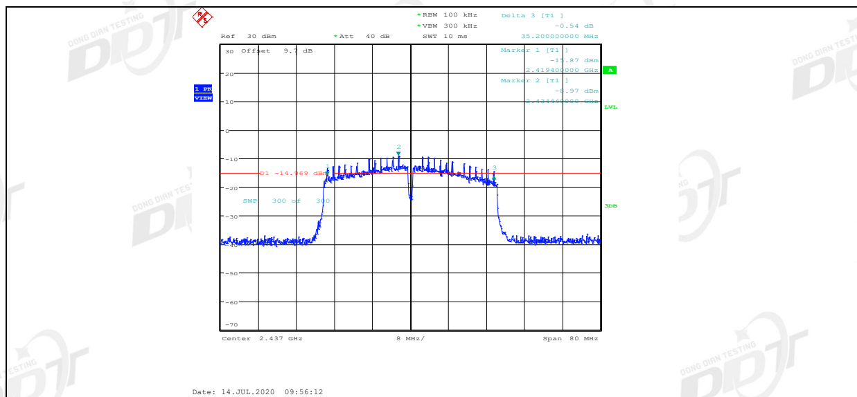
11N40MIMO Ant2 2437
