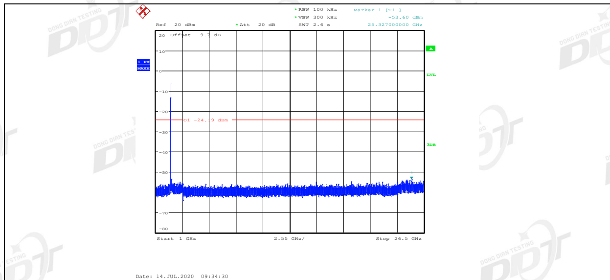
11N20MIMO_Ant2_2437_0-Reference
