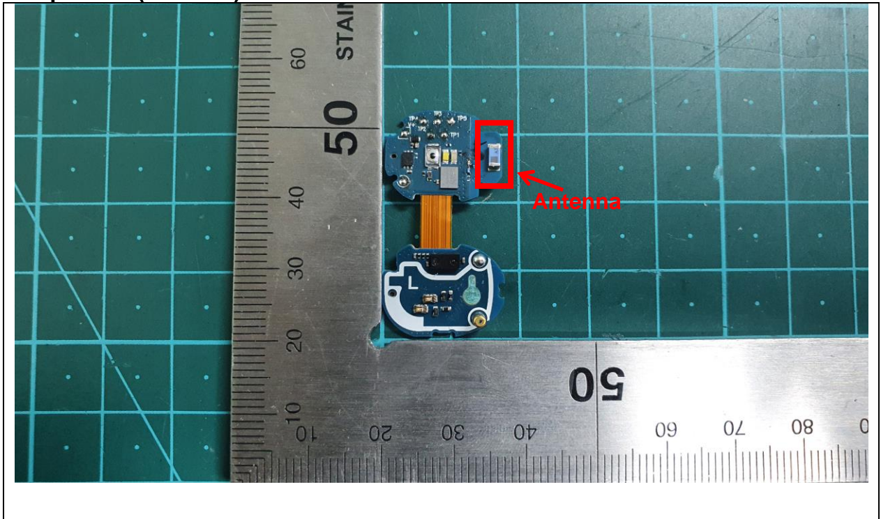
Earphone L(Antenna)
