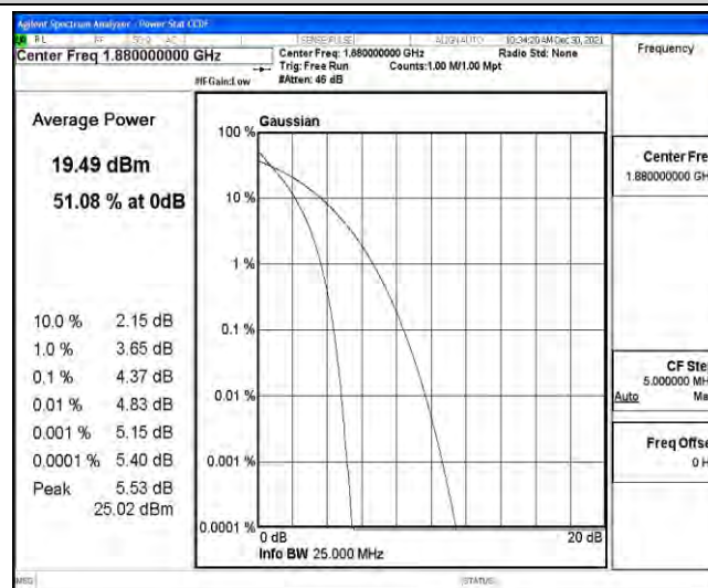
Band2-20MHz-QPSK-19100
