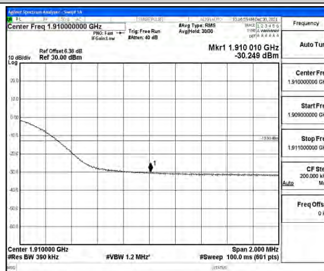
Band2-20MHz-16QAM-19100
