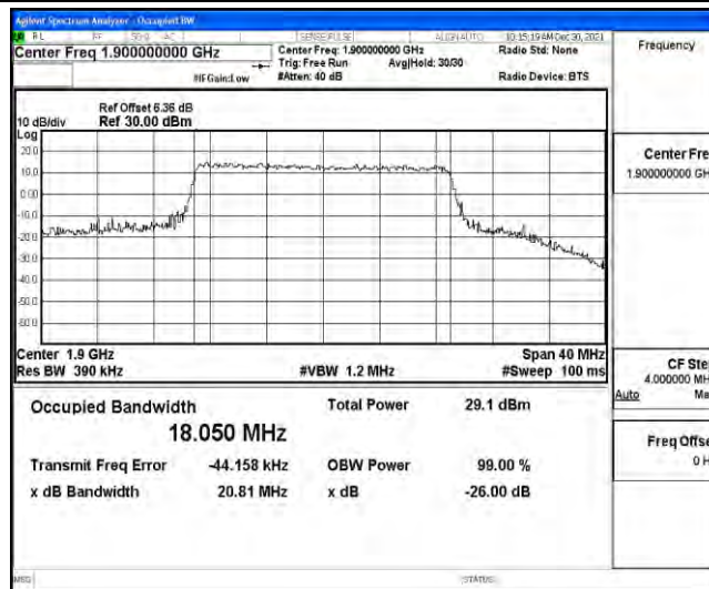
Band2-20MHz-16QAM-18700
