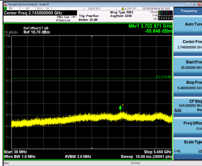
11AC80SISO_Ant2_5530_5735~40000
