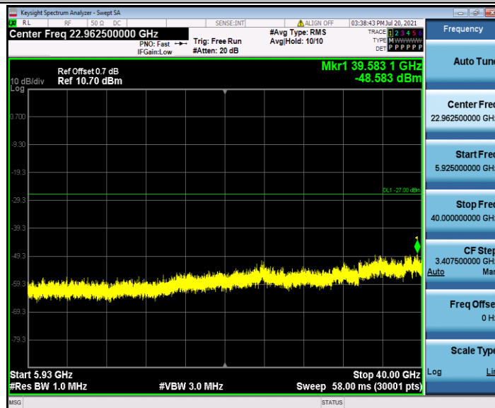
11AC80SISO_Ant1_5210_30~5140
