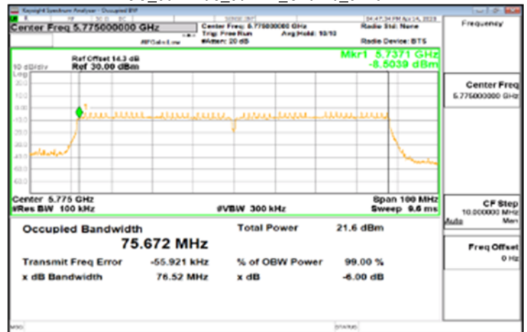
FCC_802.11ac_80MHz_Chain0_5775MHz
