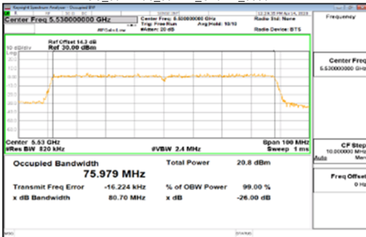
FCC_802.11ac_80MHz_Chain1_5530MHz
