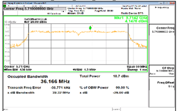
FCC_802.11n_40MHz_Chain0_5710MHz
