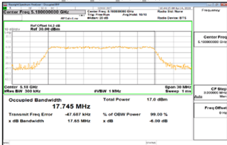
IC_802.11n_20MHz_Chain0_5180MHz
