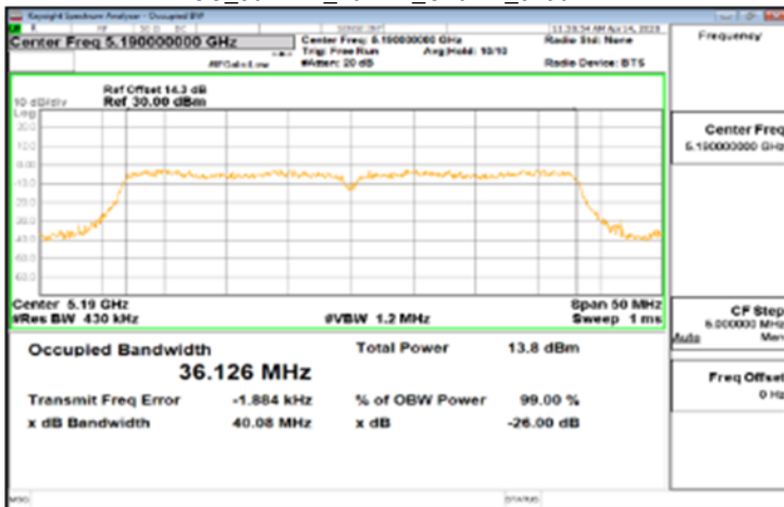
FCC_802.11n_40MHz_Chain1_5190MHz
