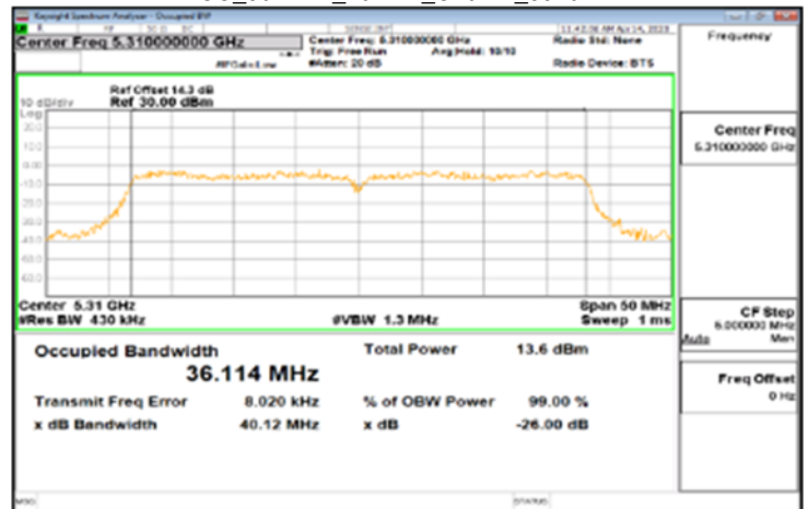
FCC_802.11n_40MHz_Chain1_5310MHz
