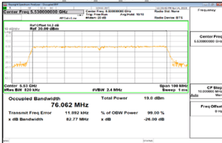
FCC_802.11ac_80MHz_Chain0_5530MHz
