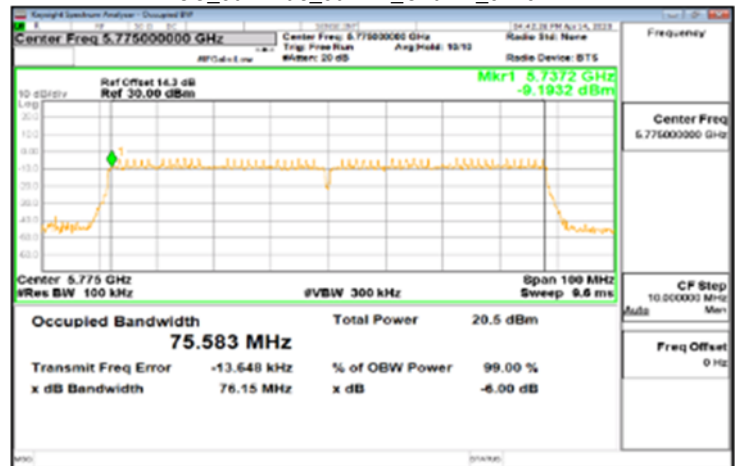
FCC_802.11ac_80MHz_Chain1_5775MHz
