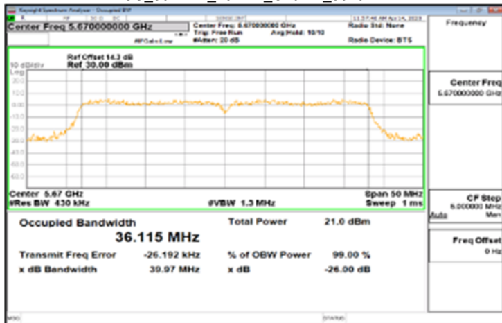
FCC_802.11n_40MHz_Chain1_5670MHz
