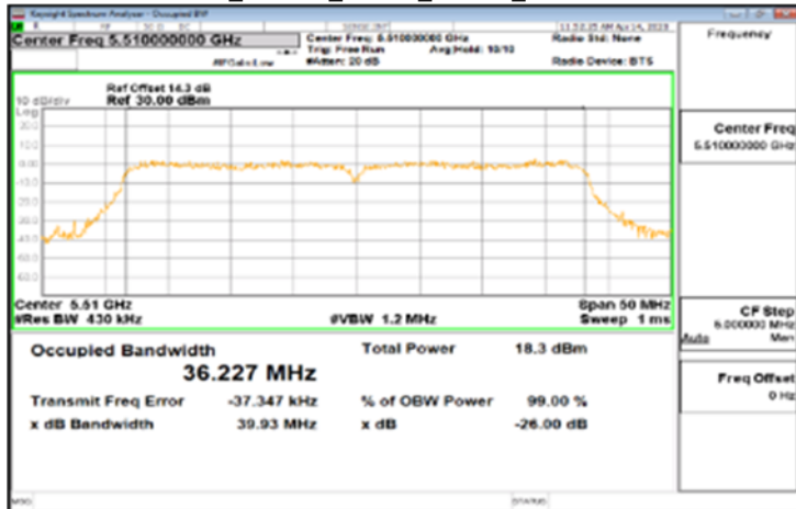
FCC_802.11n_40MHz_Chain0_5510MHz
