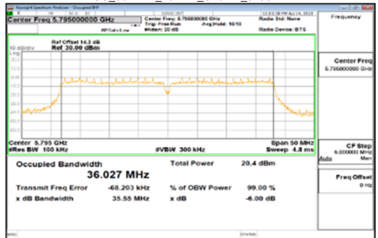
FCC_802.11n_40MHz_Chain1_5795MHz
