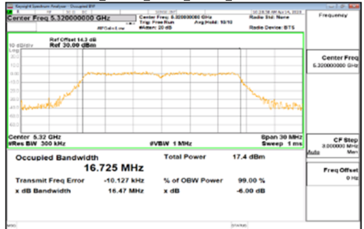
IC_802.11a_20MHz_Chain0_5320MHz
