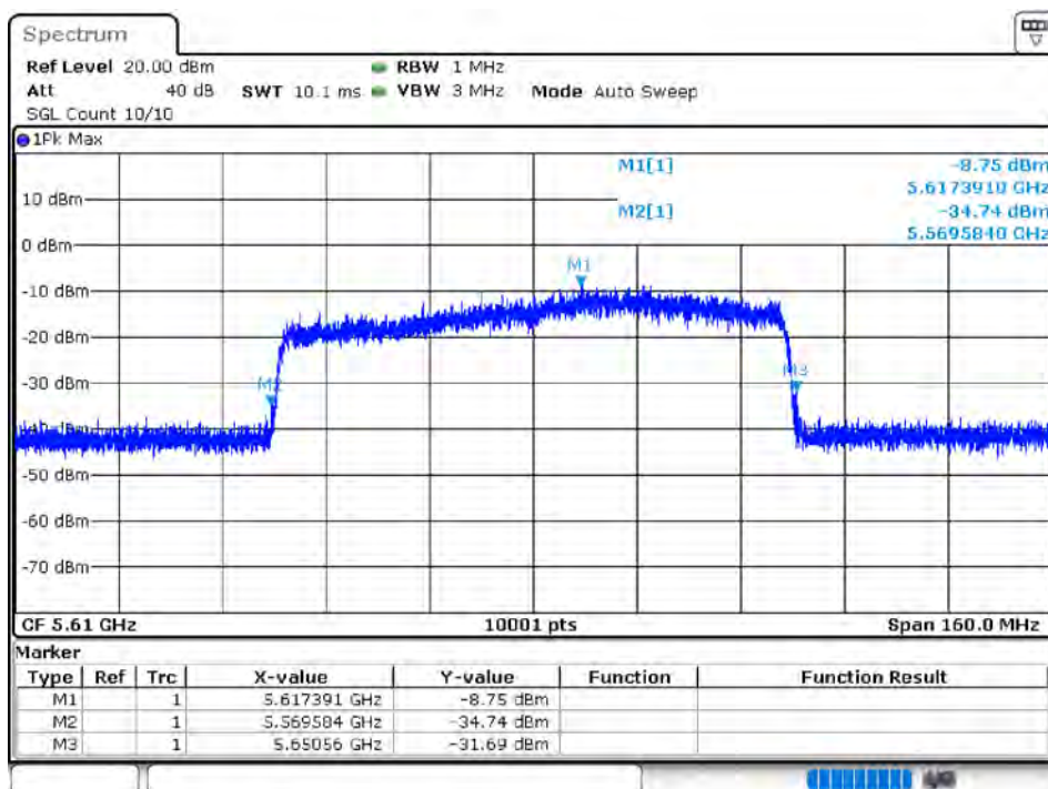
-26 dB BW NVNT 802.11ax80 5610MHz Ant 2
