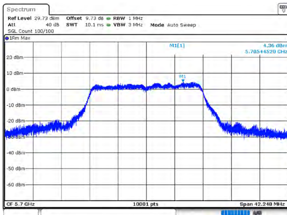
NVNT 802.11a 5700MHz Ant 1
