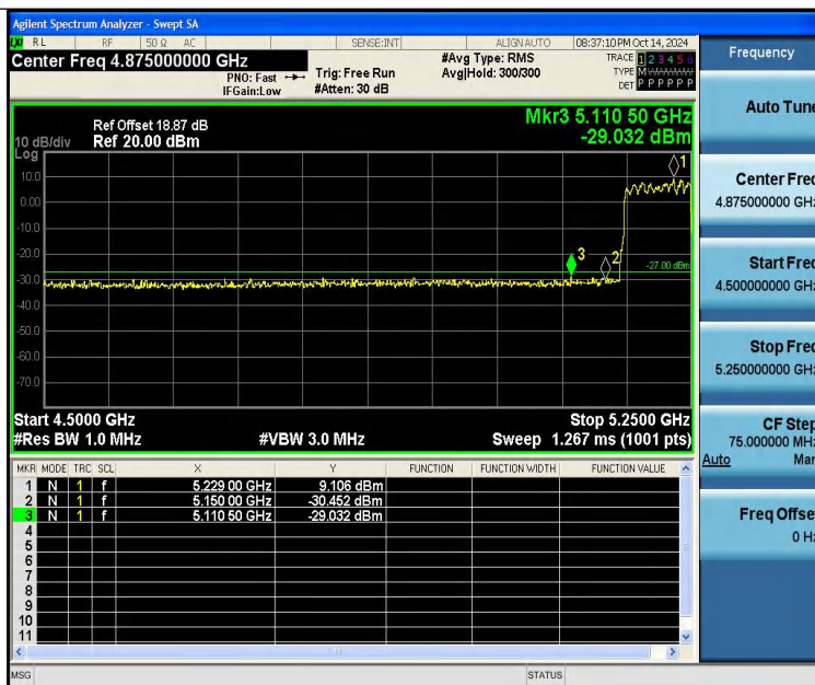
11AC80SISO-Ant1-5210-PASS
