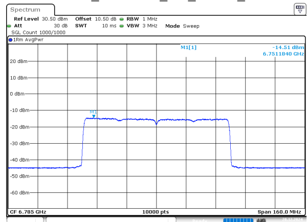
802.11ax80_6785MHz_RU_996/67_Chain 2
