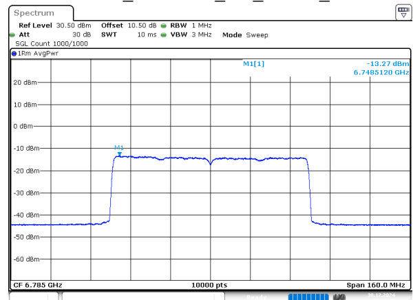
802.11ax80_6785MHz_RU_996/67_Chain 1
