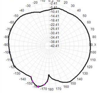
2400.0MHz Total(E1-XZ), Max=-2.81dBi
