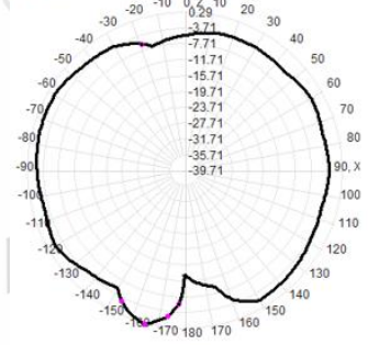
2480.0MHz Total(E1-XZ), Max=0.29dBi
