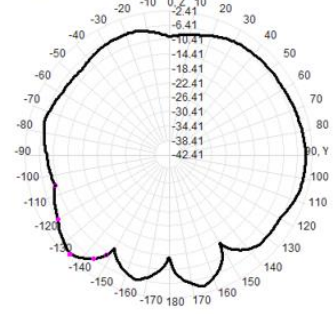
2400.0MHz Total(E2-YZ), Max=-3.54dBi
