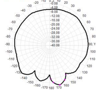
2480.0MHz Total(E2-YZ), Max=-1.66dBi
