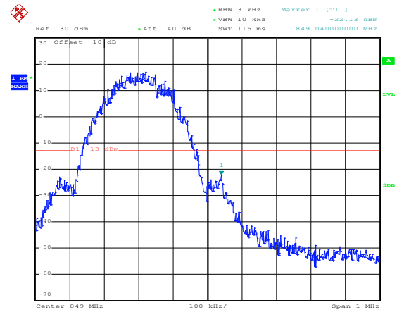
EGPRS850
