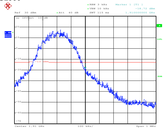
EGPRS1900
