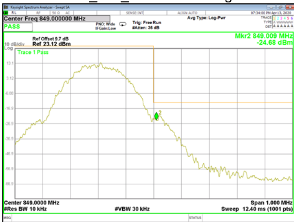
GSM_850_Higher_Band edge
