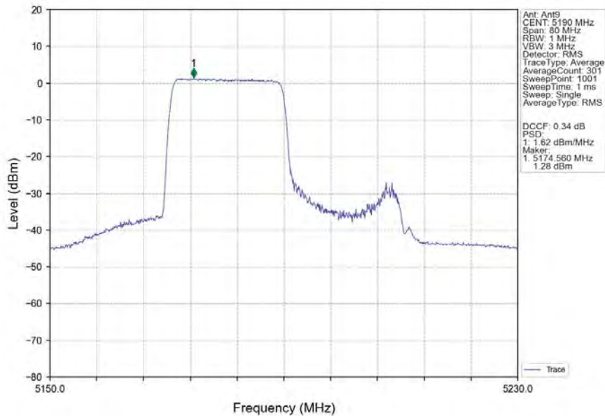
802.11ax(HEW40)_LCH_5190MHz_RU242_Left_Ant9_NTNV
