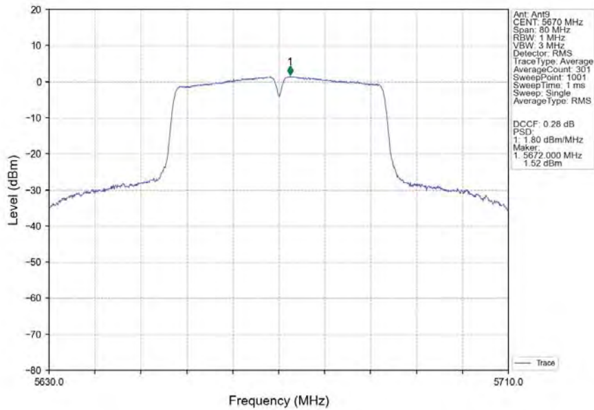
802.11n(HT40)_HCH_5670MHz_Ant9_NTNV
