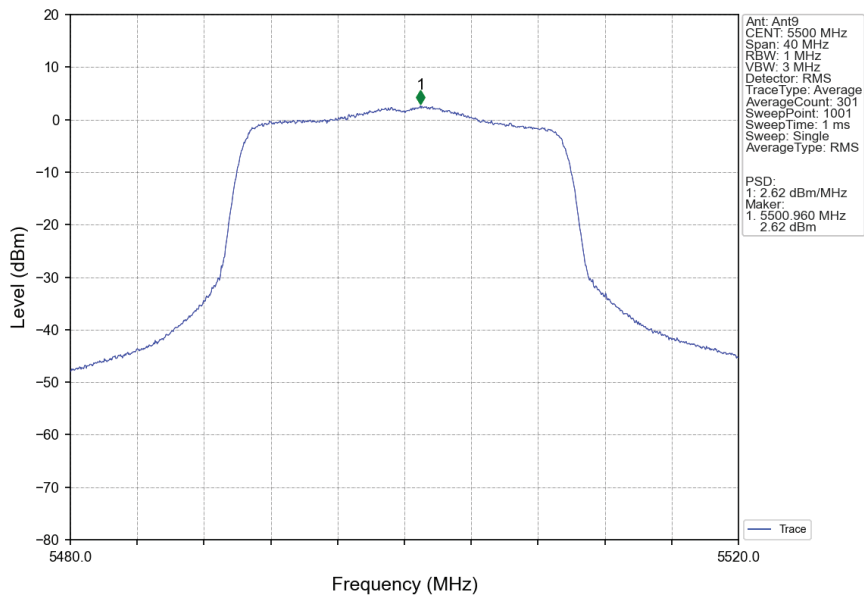
802.11ax(HEW20)_LCH_5500MHz_RU242_Left_Ant9_NTNV
