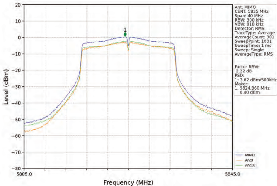
802.11n(HT20)_HCH_5825MHz_MIMO_NTNV
