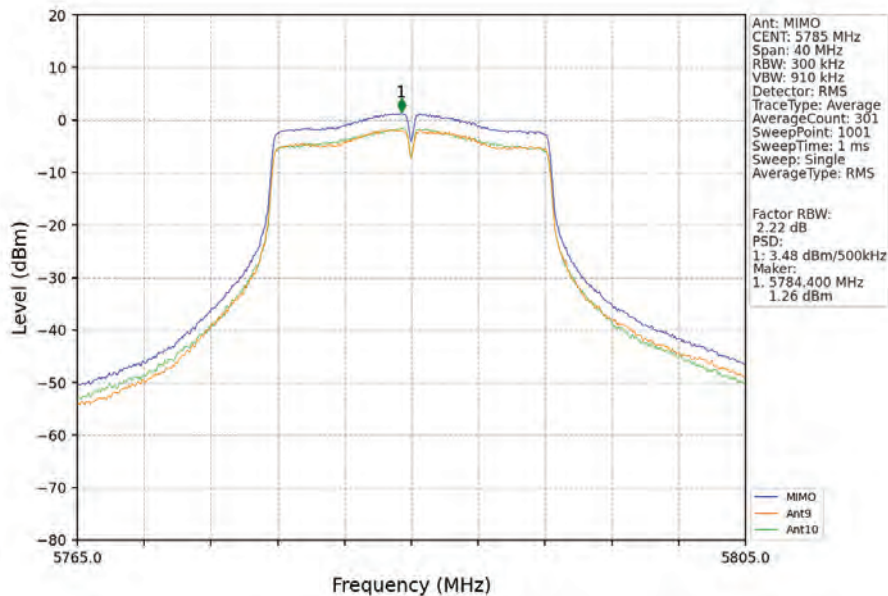
802.11a_MCH_5785MHz_MIMO_NTNV
