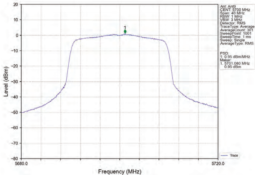
802.11ax(HEW20)_HCH_5700MHz_RU242_Left_Ant9_NTNV
