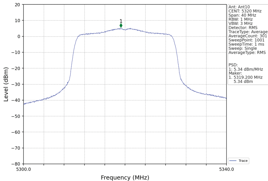
802.11ax(HEW20)_HCH_5320MHz_RU242_Left_Ant10_NTNV
