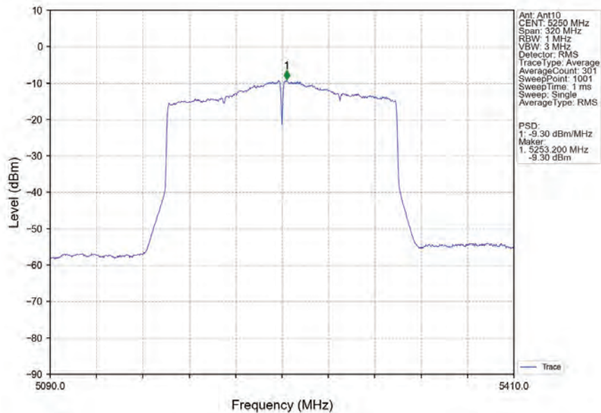
802.11ax(HEW160)_MCH_5250MHz_2xRU996_Left_Ant10_NTNV
