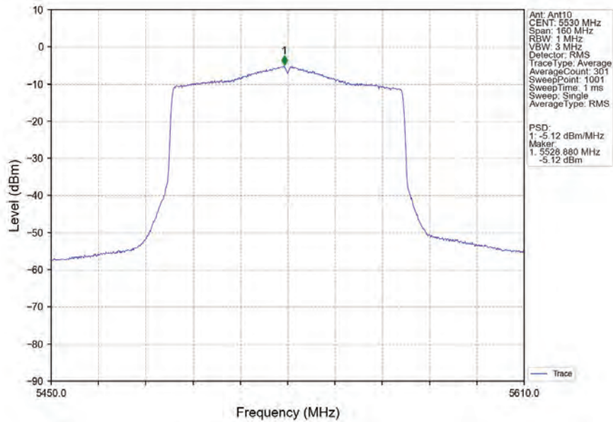
802.11ax(HEW80)_LCH_5530MHz_RU996_Left_MIMO_NTNV
