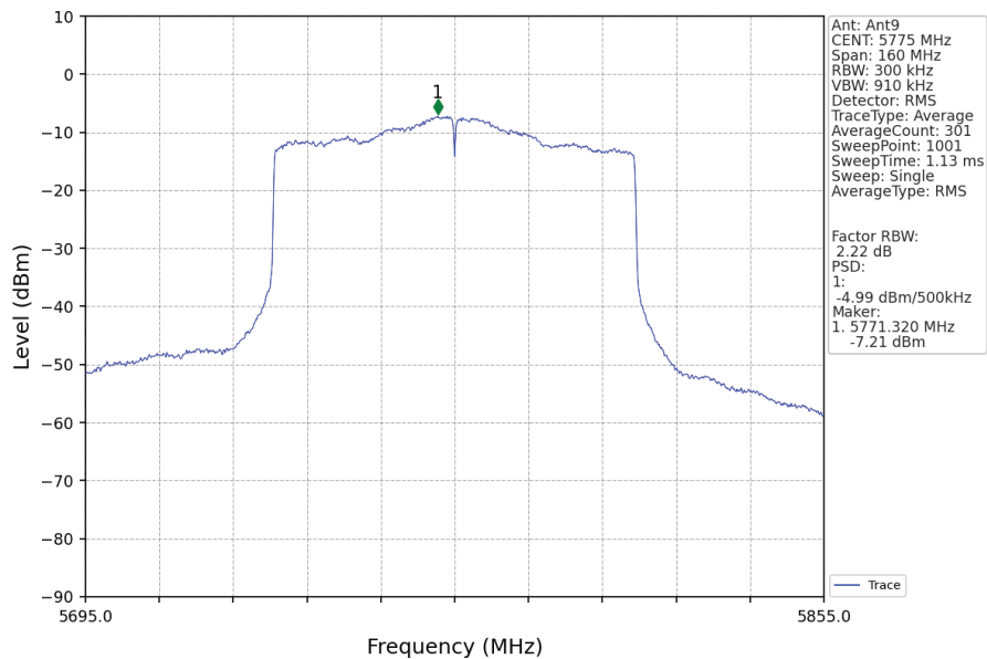
802.11ax(HEW80)_MCH_5775MHz_RU996_Left_Ant9_NTNV
