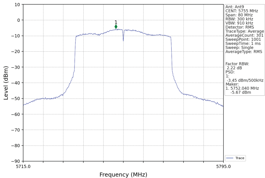
802.11ax(HEW40)_LCH_5755MHz_RU484_Left_Ant9_NTNV
