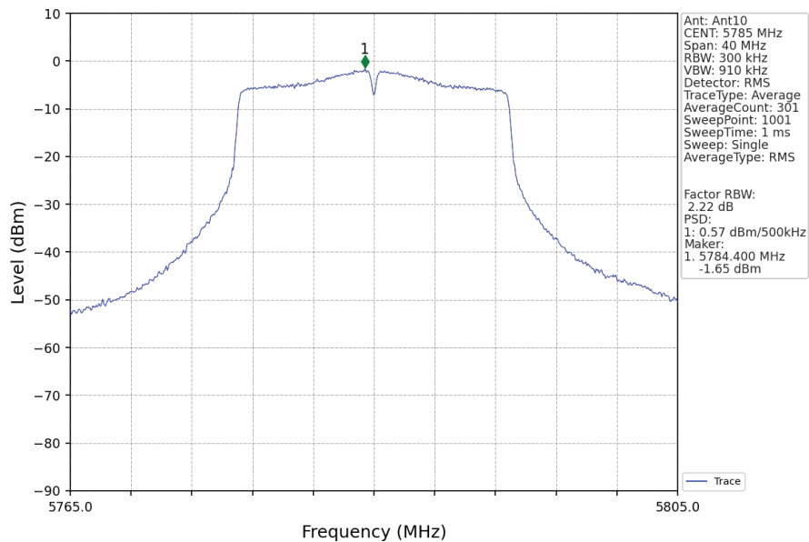
802.11n(HT20)_MCH_5785MHz_Ant10_NTNV
