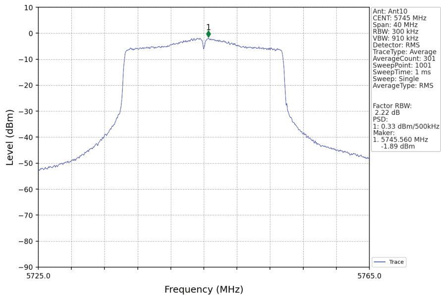
802.11ax(HEW20)_LCH_5745MHz_RU242_Left_Ant10_NTNV
