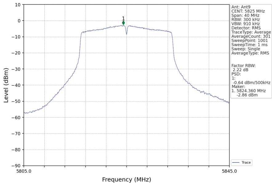
802.11n(HT20)_HCH_5825MHz_Ant9_NTNV
