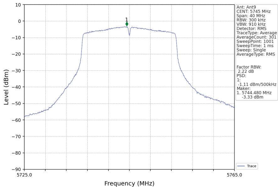
802.11n(HT20)_LCH_5745MHz_Ant9_NTNV
