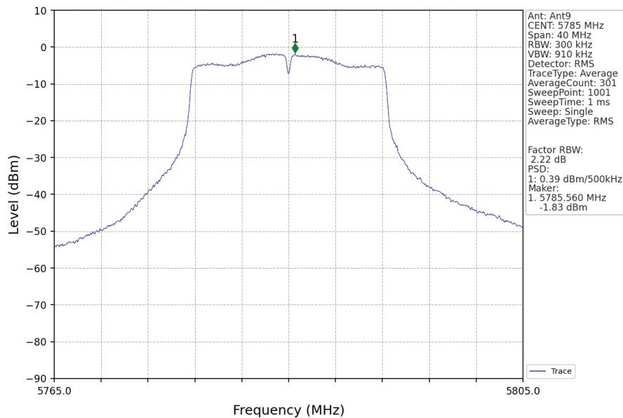
802.11a_MCH_5785MHz_Ant9_NTNV
