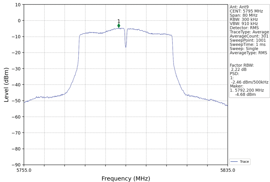
802.11n(HT40)_HCH_5795MHz_Ant9_NTNV
