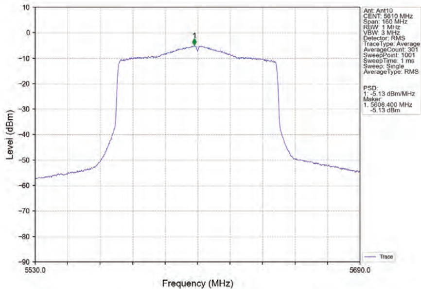
802.11ax(HEW80)_HCH_5610MHz_RU996_Left_Ant10_NTNV
