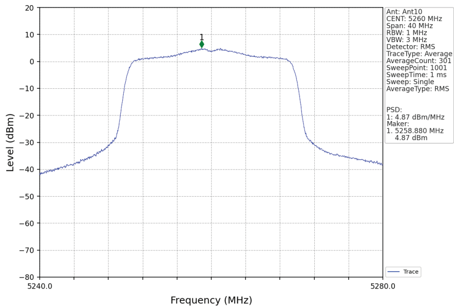
802.11ax(HEW20)_LCH_5260MHz_RU242_Left_Ant10_NTNV
