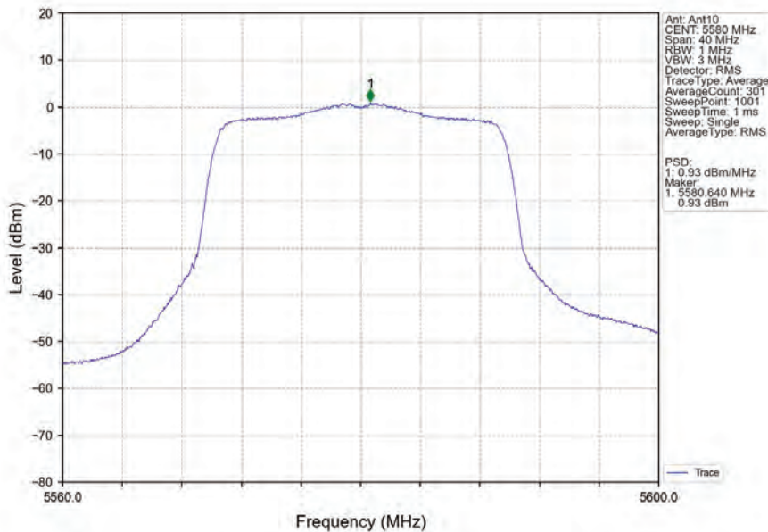
802.11ax(HEW20)_MCH_5580MHz_RU242_Left_Ant10_NTNV
