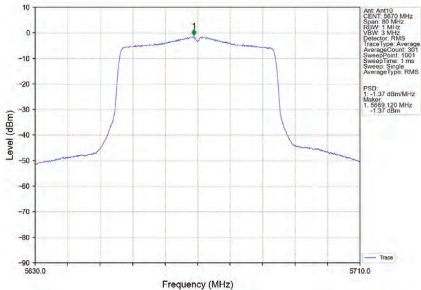
802.11ax(HEW40)_HCH_5670MHz_RU484_Left_Ant10_NTNV
