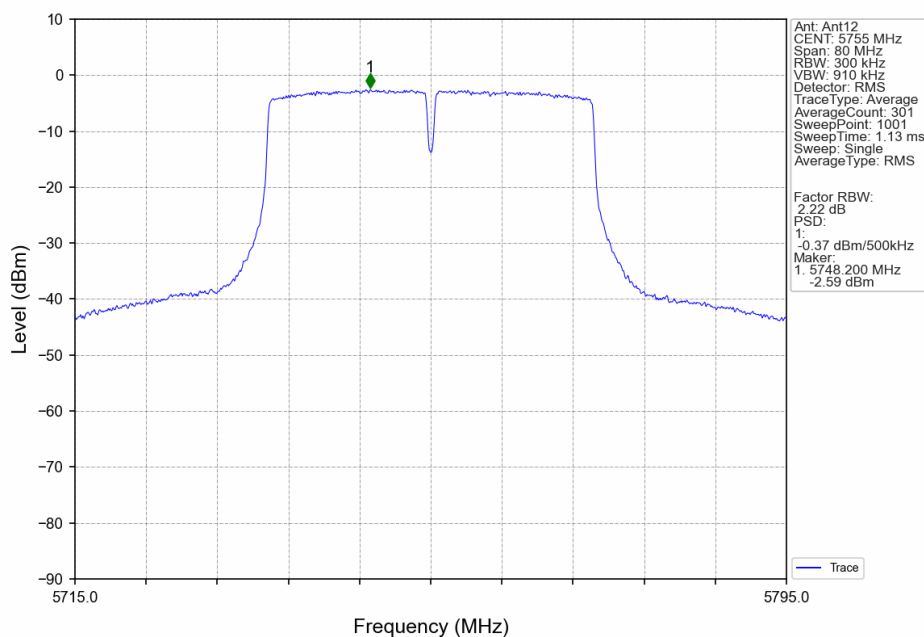
802.11ac(VHT40)_LCH_5755MHz_Ant12_NTNV
