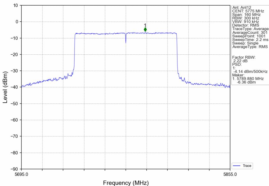
802.11ax(HEW80)_MCH_5775MHz_RU996_Left_Ant12_NTNV
