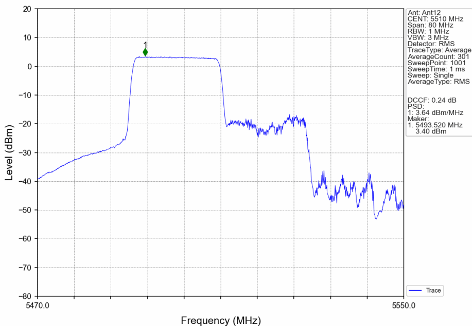
802.11ax(HEW40)_LCH_5510MHz_RU242_Left_Ant12_NTNV
