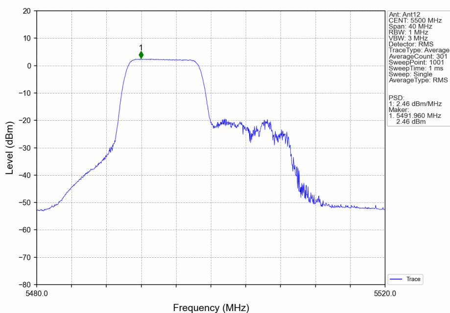
802.11ax(HEW20)_LCH_5500MHz_RU106_Left_Ant12_NTNV
