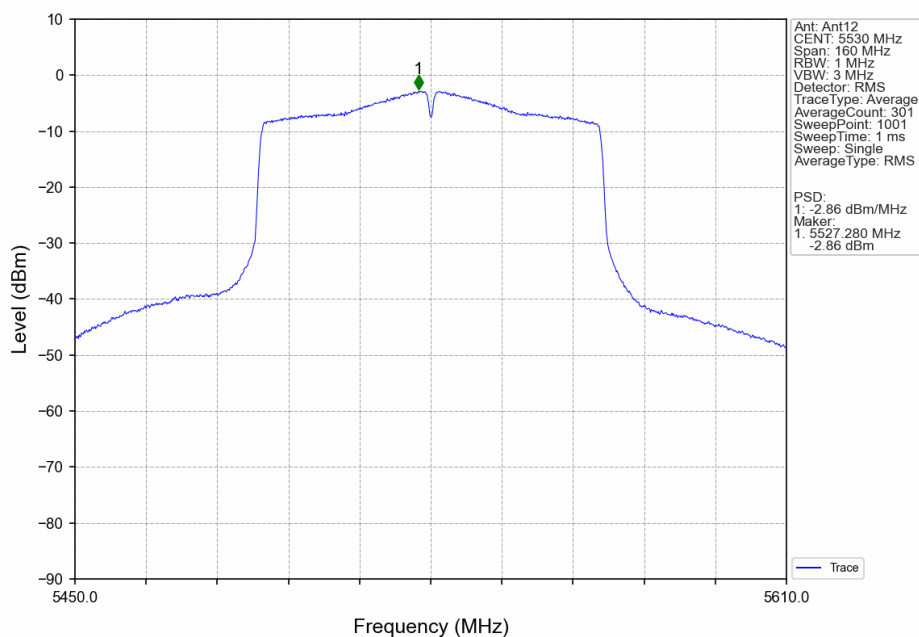
802.11ac(VHT80)_LCH_5530MHz_Ant12_NTNV
