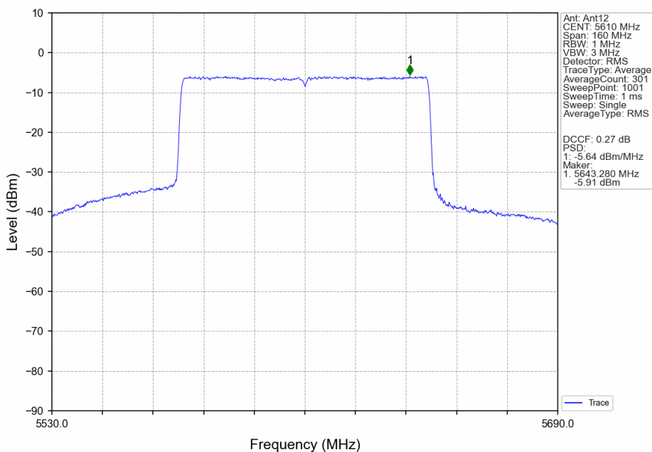
802.11ax(HEW80)_HCH_5610MHz_RU996_Left_Ant12_NTNV
