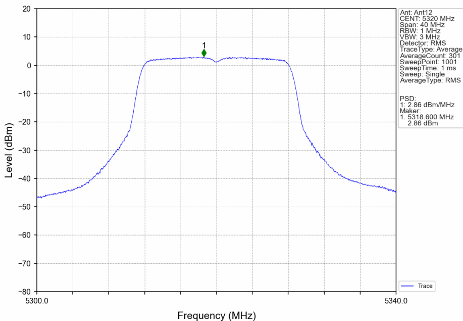
802.11a_HCH_5320MHz_Ant12_NTNV
