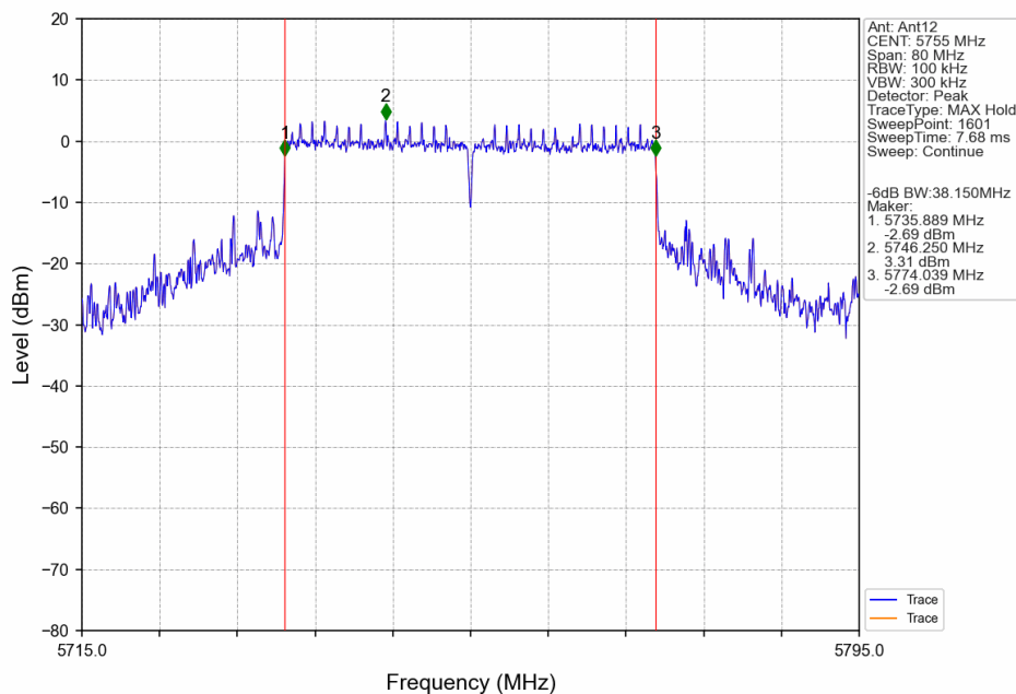
802.11ax(HEW40)_LCH_5755MHz_RU484_Left_Ant12_NTNV
