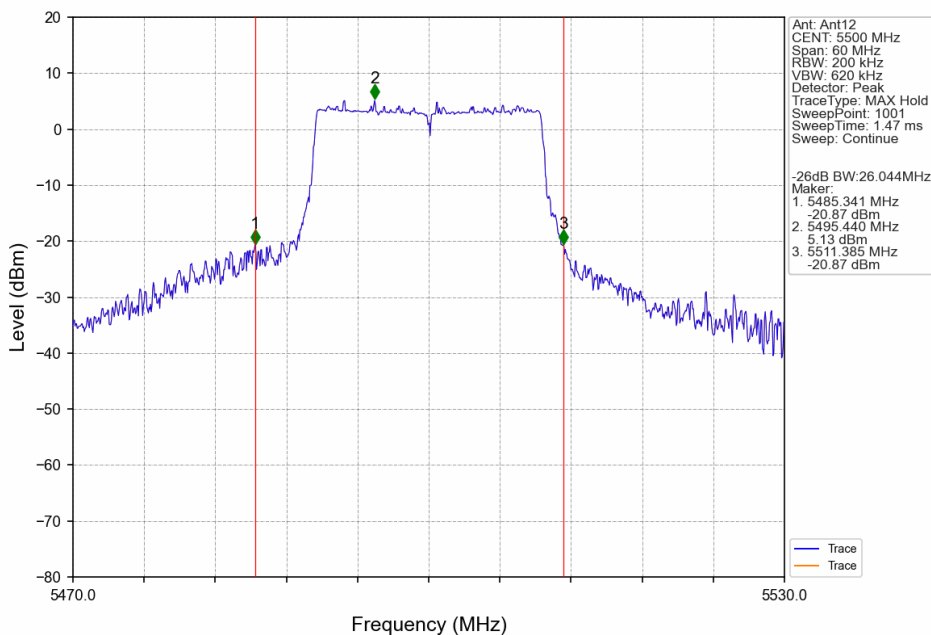
802.11ax(HEW20)_LCH_5500MHz_RU242_Left_Ant12_NTNV
