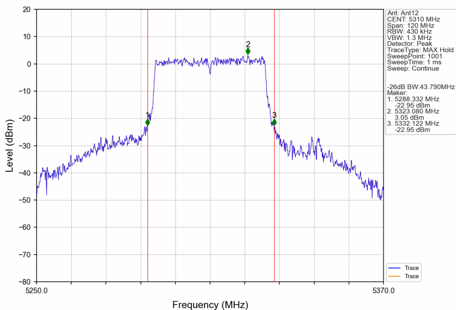
802.11ax(HEW40)_HCH_5310MHz_RU484_Left_Ant12_NTNV
