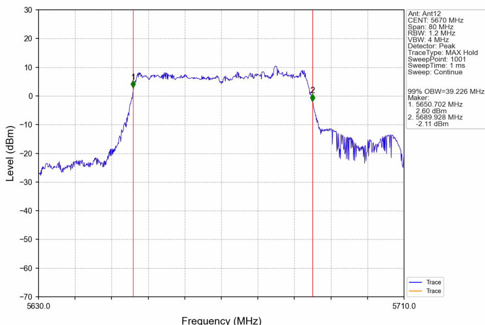
802.11ax(HEW40)_HCH_5670MHz_RU484_Left_Ant12_NTNV
