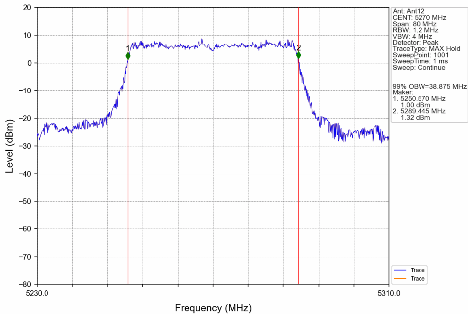
802.11ax(HEW40)_LCH_5270MHz_RU484_Left_Ant12_NTNV
