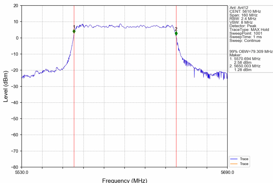
802.11ax(HEW80)_HCH_5610MHz_RU996_Left_Ant12_NTNV
