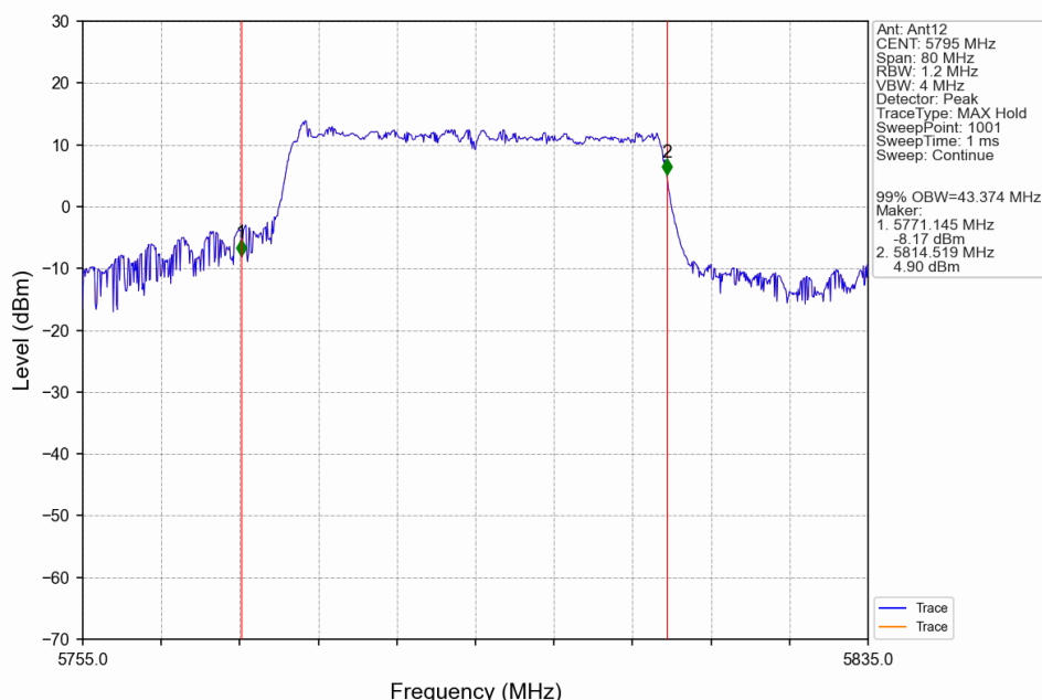
802.11ax(HEW40)_HCH_5795MHz_RU484_Left_Ant12_NTNV
