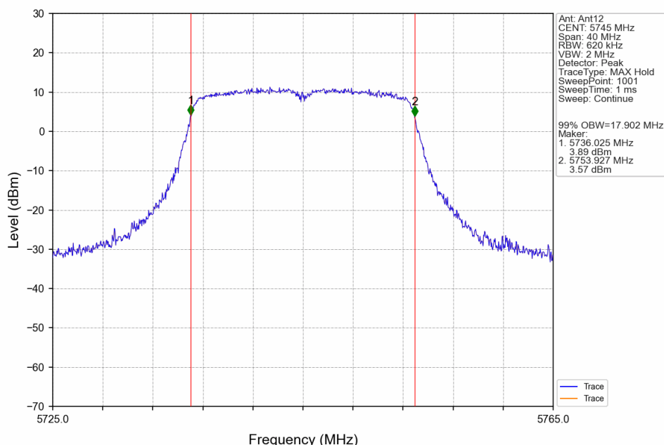
802.11n(HT20)_LCH_5745MHz_Ant12_NTNV
