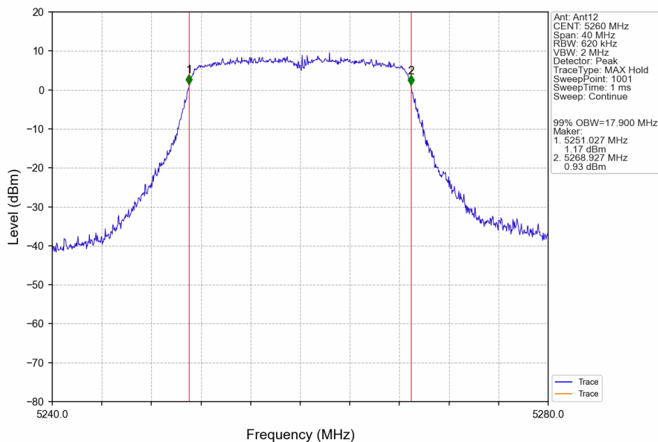
802.11n(HT20)_LCH_5260MHz_Ant12_NTNV
