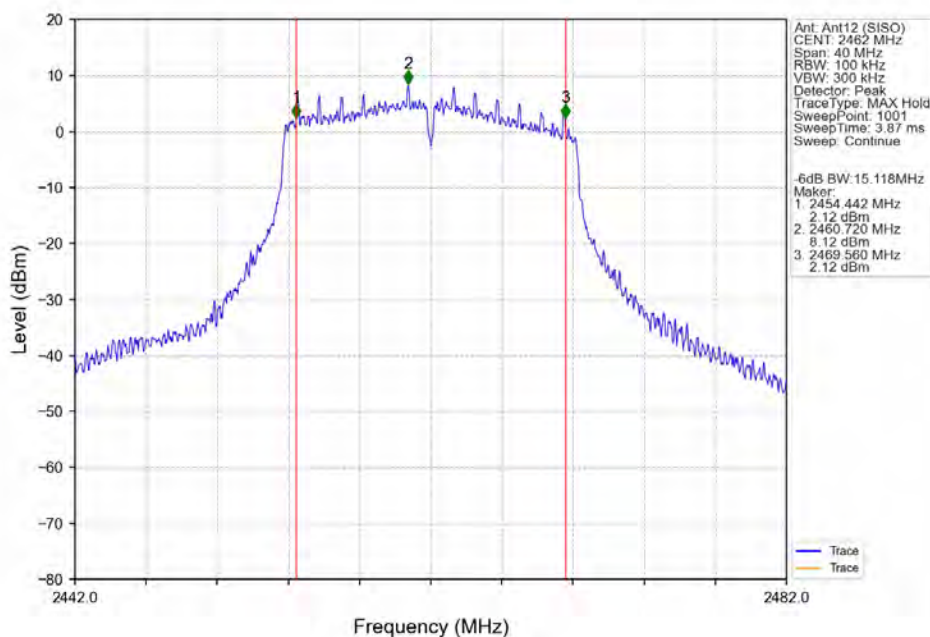
802.11g_HCH_2462MHz_Ant12 (SISO)_NTNV
