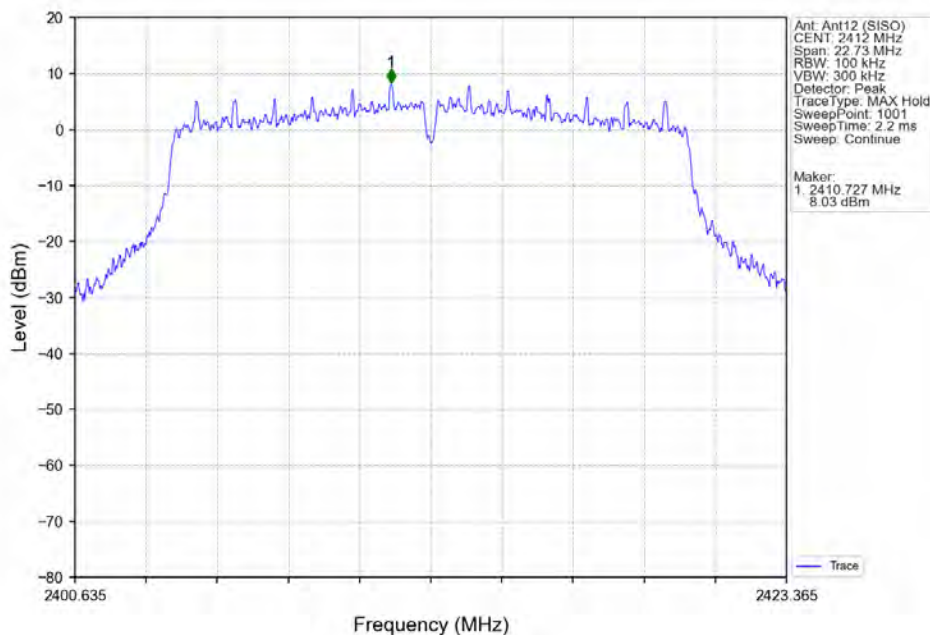
802.11g_LCH_2412MHz_Ant12 (SISO)_NTNV
