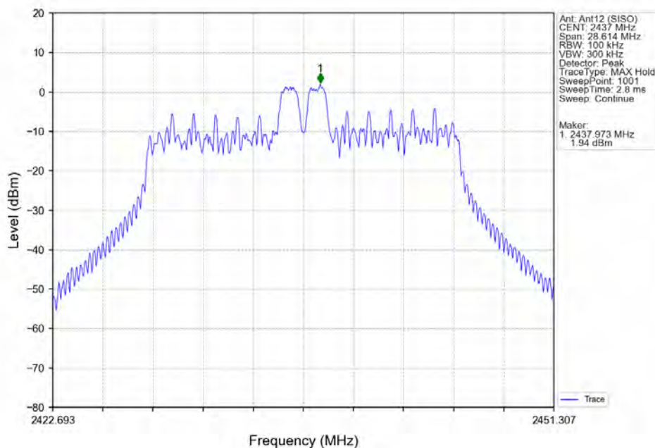
802.11ax(HEW20)_MCH_2437MHz_RU52_Mid_Ant12 (SISO)_NTNV
