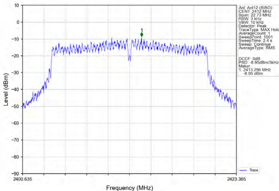
802.11g_LCH_2412MHz_Ant12 (SISO)_NTNV
