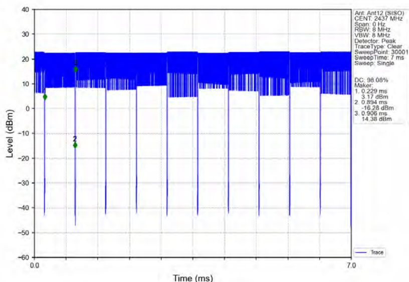
802.11b_MCH_2437MHz_Ant12 (SISO)_NTNV
