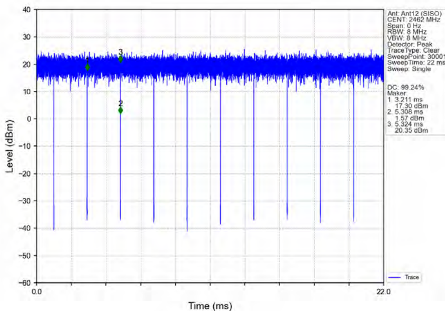
802.11g_HCH_2462MHz_Ant12 (SISO)_NTNV
