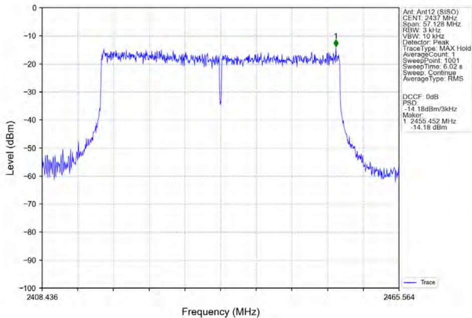
802.11ax(HEW40)_MCH_2437MHz_RU484_Left_Ant12 (SISO)_NTNV
