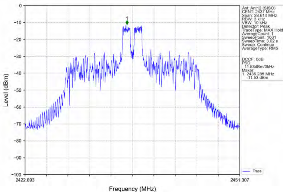
802.11ax(HEW20)_MCH_2437MHz_RU52_Mid_Ant12 (SISO)_NTNV
