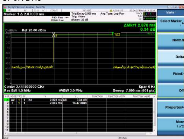
GFSK DH5
