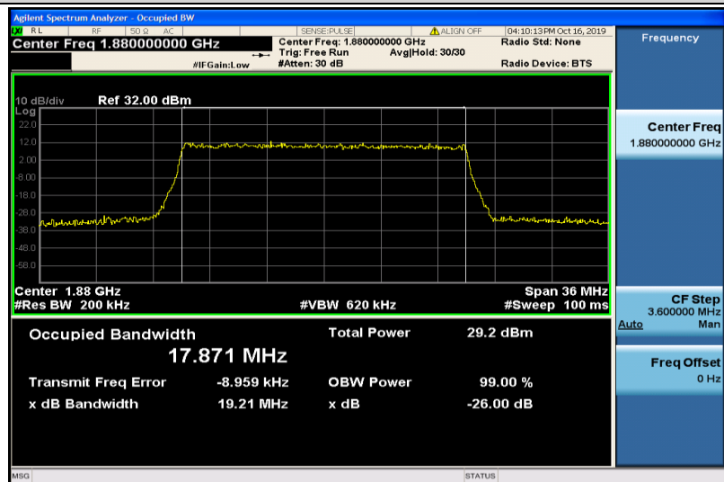
Band2-20MHz-QPSK-18900-100RB#0-17.871
