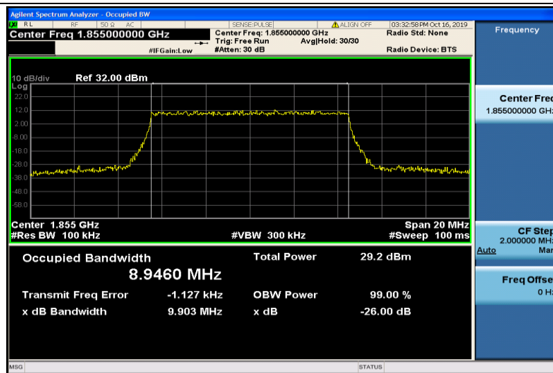
Band2-10MHz-QPSK-18650-50RB#0-8.9460
