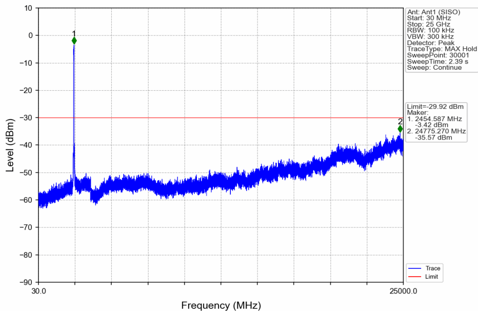
802.11n(HT40)_HCH_2452MHz_Ant1 (SISO)_NTNV
