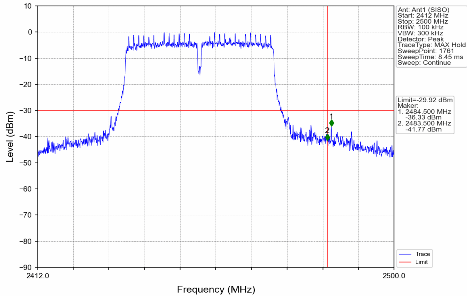
802.11n(HT40)_HCH_2452MHz_Ant1 (SISO)_NTNV
