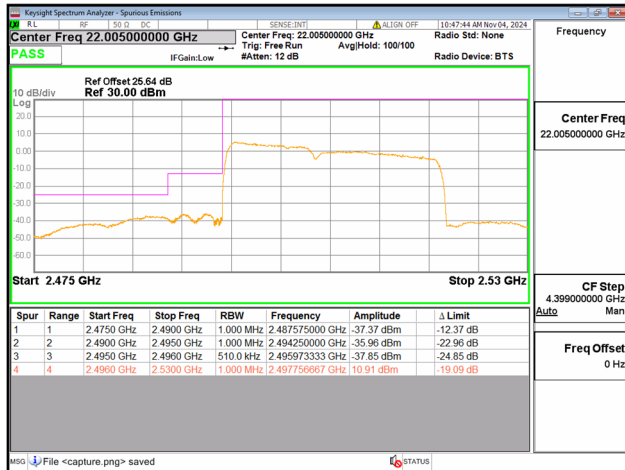
41C / 10+15MHz / Low CH / QPSK / 50#0-75#0
