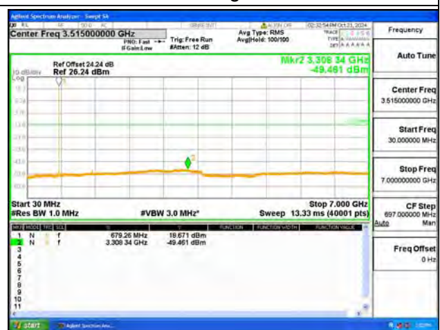
B71 / 20MHz / High CH / 64QAM
