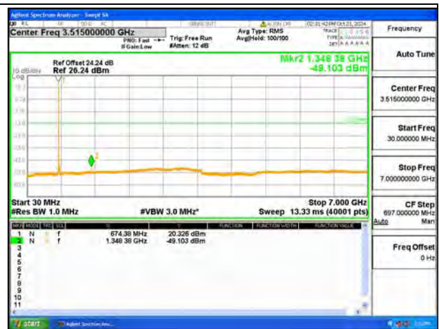
B71 / 20MHz / Mid CH / 16QAM
