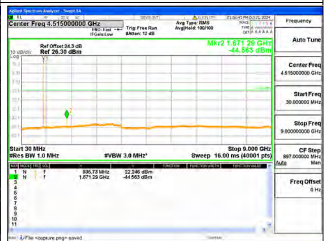
B19 / 10MHz / High CH / QPSK
