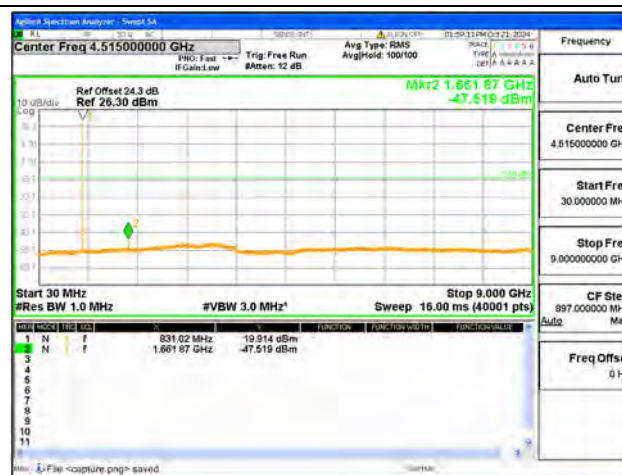
B19 / 15MHz / Mid CH / 64QAM
