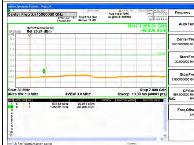
B71 / 5MHz / Mid CH / 16QAM
