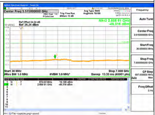
B71 / 15MHz / Mid CH / 64QAM
