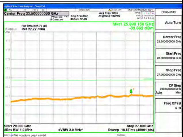
B41-20G-27G / 20MHz / High CH / QPSK
