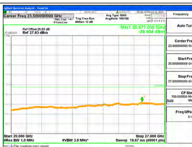
B41-20G-27G / 5MHz / Low CH / QPSK
