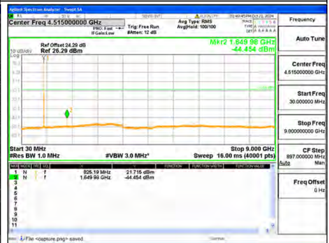
B18 part22 / 5MHz / Mid CH / QPSK
