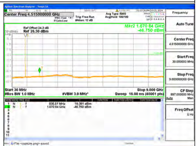
B19 / 5MHz / Mid CH / 64QAM
