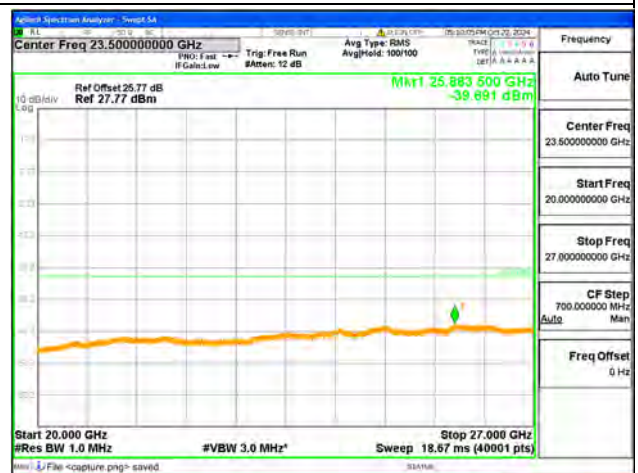
B41-20G-27G / 10MHz / High CH / QPSK
