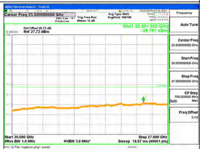
B38-20G-27G / 15MHz / High CH / QPSK
