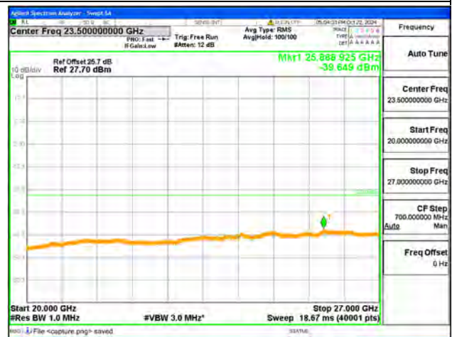
B38-20G-27G / 20MHz / Mid CH / QPSK
