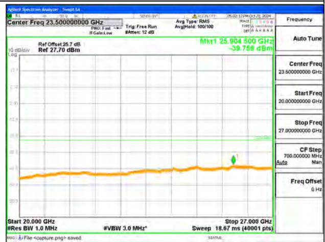
B38-20G-27G / 15MHz / Mid CH / QPSK
