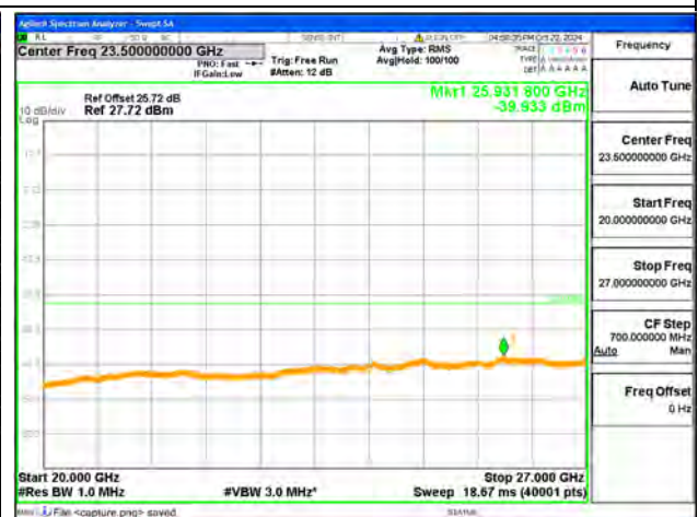
B38-20G-27G / 5MHz / High CH / QPSK
