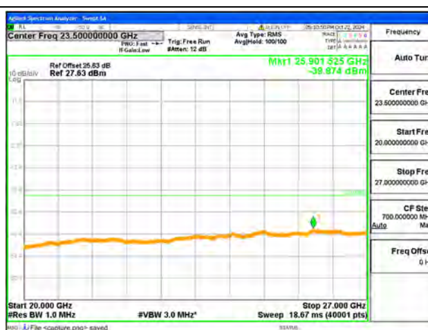
B41-20G-27G / 15MHz / Low CH / QPSK
