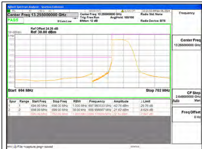
B12 / 1.4MHz / Low CH / QPSK / 1 RB
