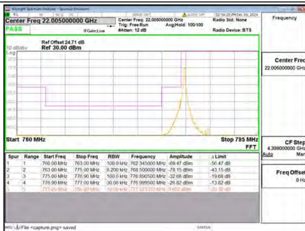
B13 / 5MHz / Low CH / QPSK / 1 RB
