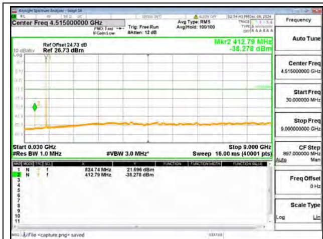
B26 / 1.4MHz / Low CH / QPSK
