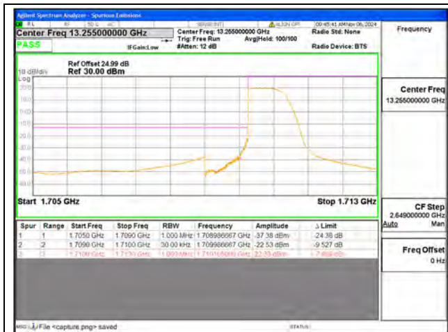
B4 / 1.4MHz / Low CH / QPSK / 1 RB
