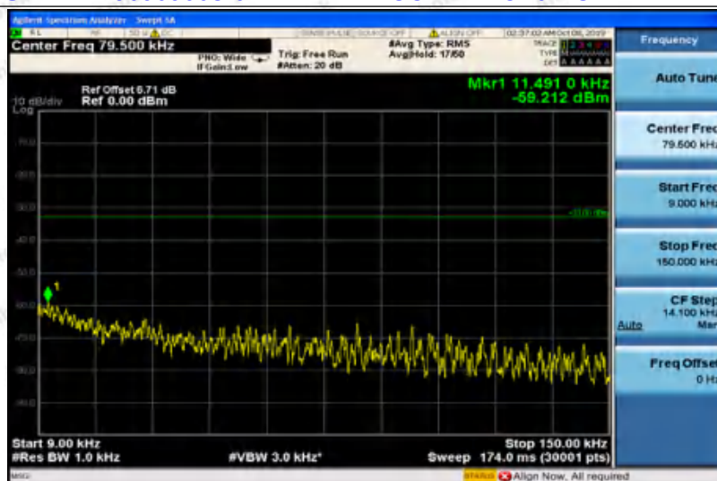
EGPRS850-128-0.009~0.15
