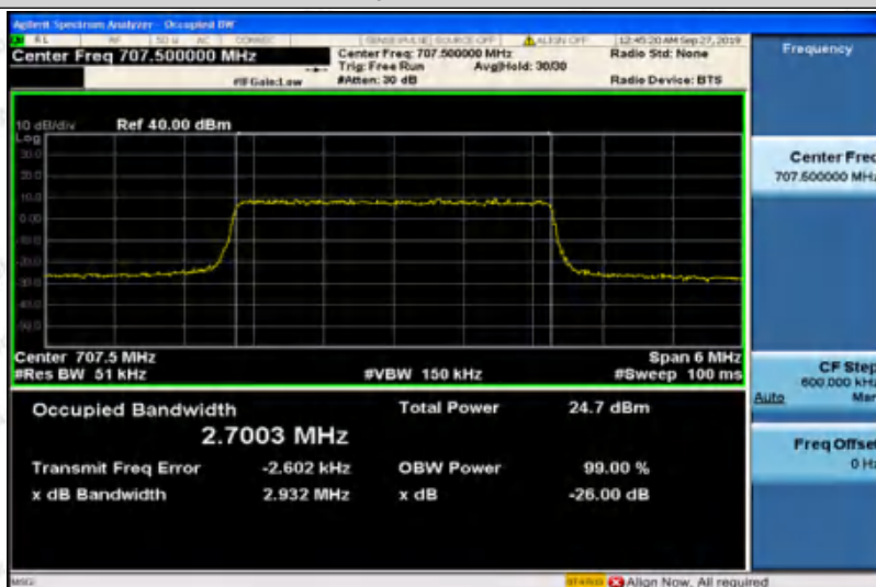
Band12-3MHz-QPSK-23165-15RB#0-2.6969
