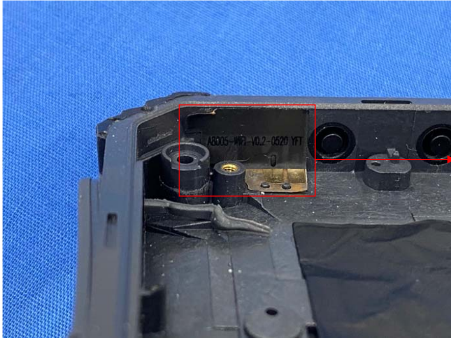
Wi-Fi/BLE/BT Antenna
