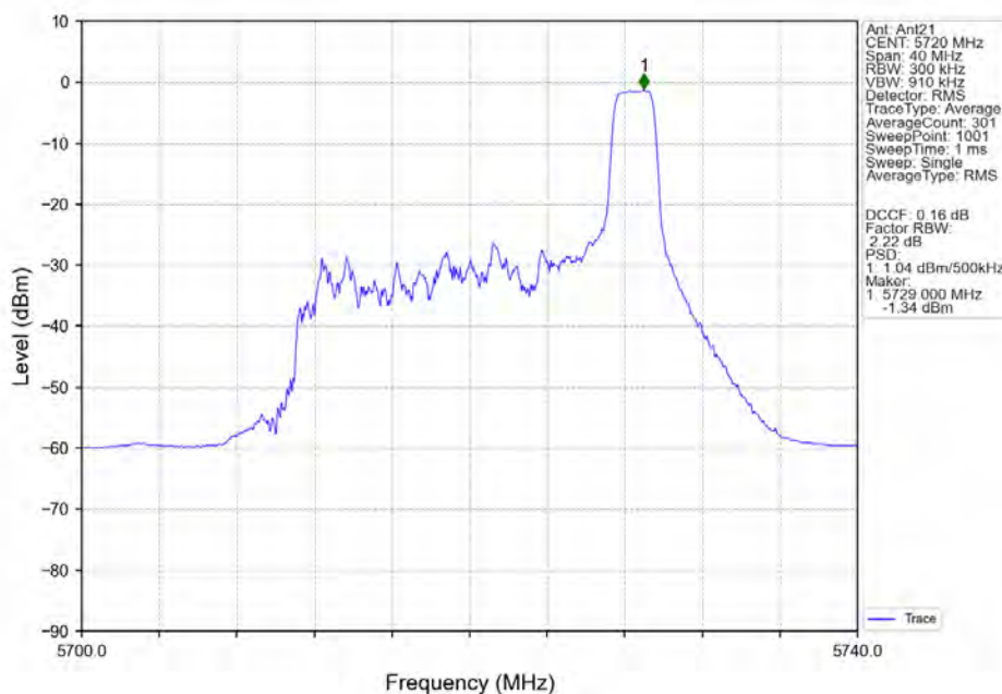
802.11ax(HEW20)_HCH_5720MHz_RU26_Right_Ant21_NTNV
