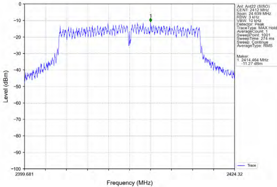
802.11g_LCH_2412MHz_Ant22 (SISO)_NTNV
