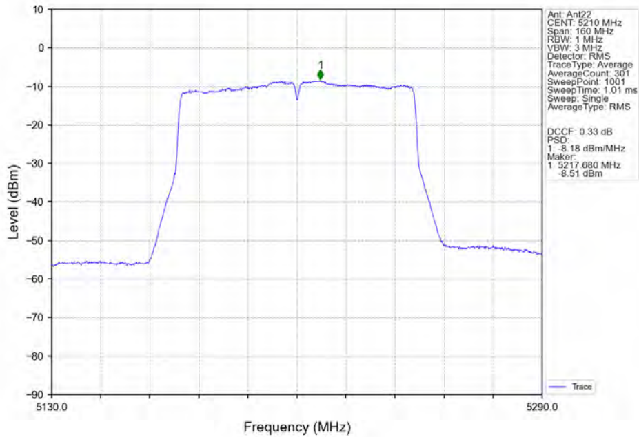
802.11ac(VHT80)_MCH_5210MHz_Ant22_NTNV
