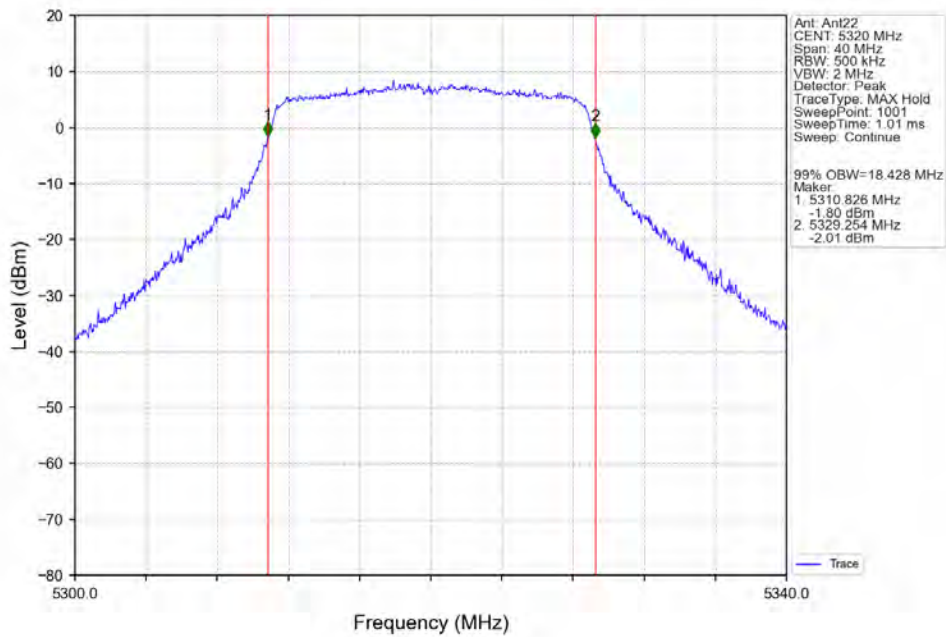
802.11n(HT20)_HCH_5320MHz_Ant22_NTNV
