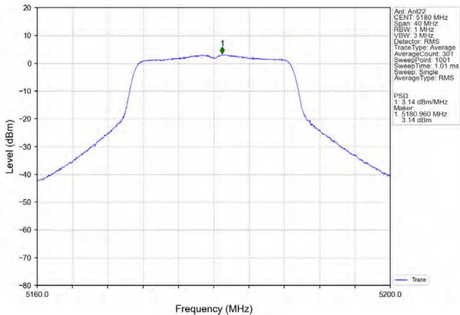
802.11n(HT20)_LCH_5180MHz_Ant22_NTNV
