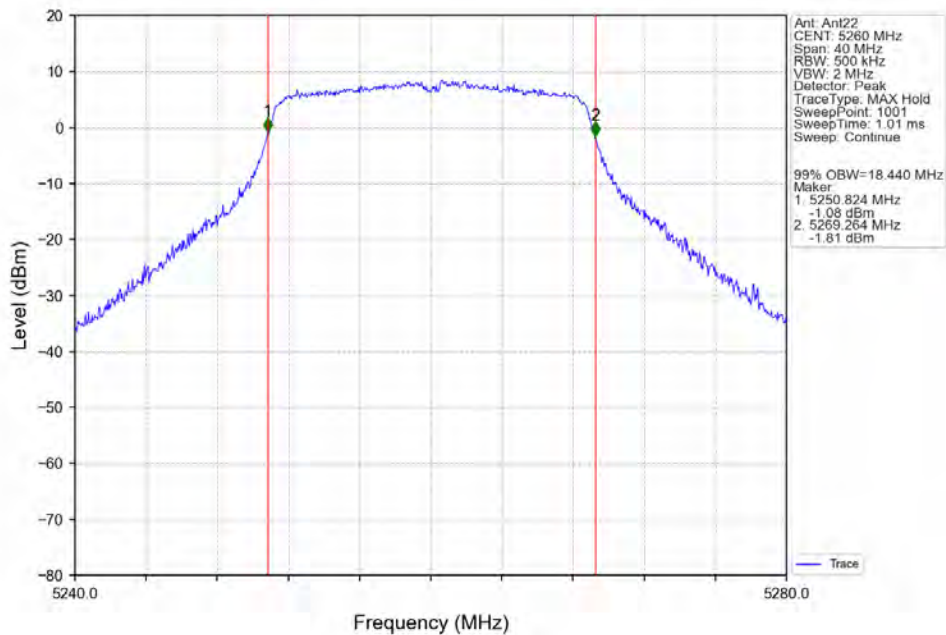
802.11n(HT20)_LCH_5260MHz_Ant22_NTNV
