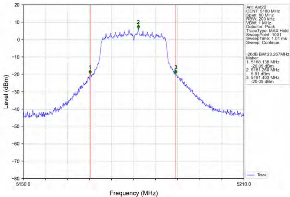
802.11n(HT20)_LCH_5180MHz_Ant22_NTNV
