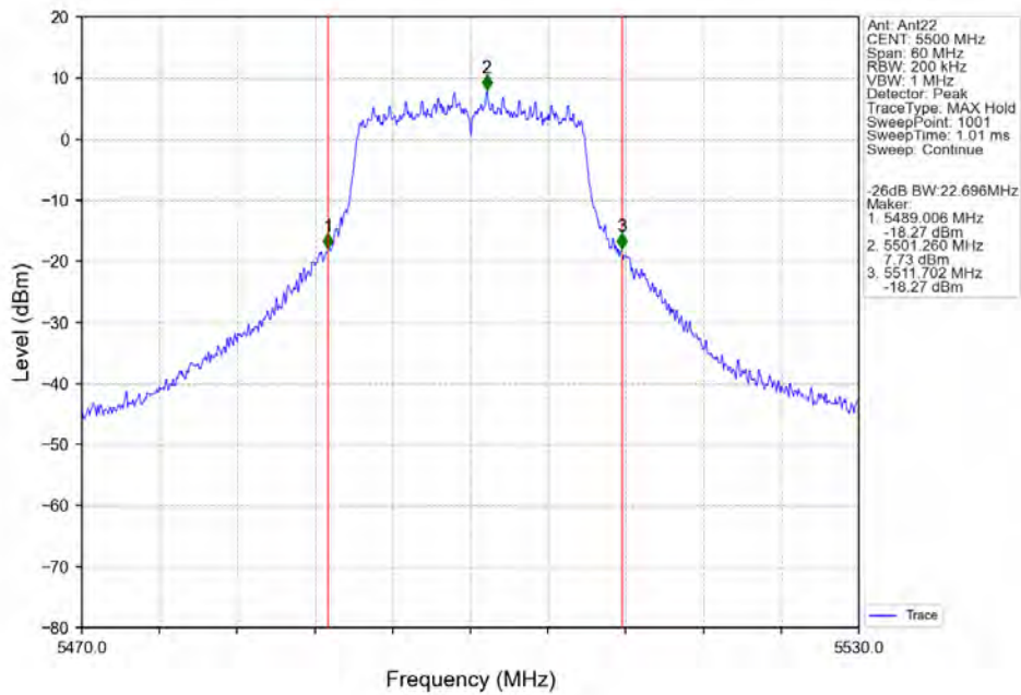
802.11n(HT20)_LCH_5500MHz_Ant22_NTNV
