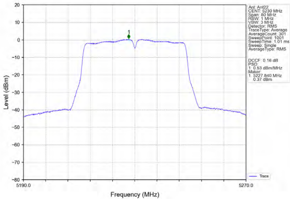
802.11n(HT40)_HCH_5230MHz_Ant22_NTNV
