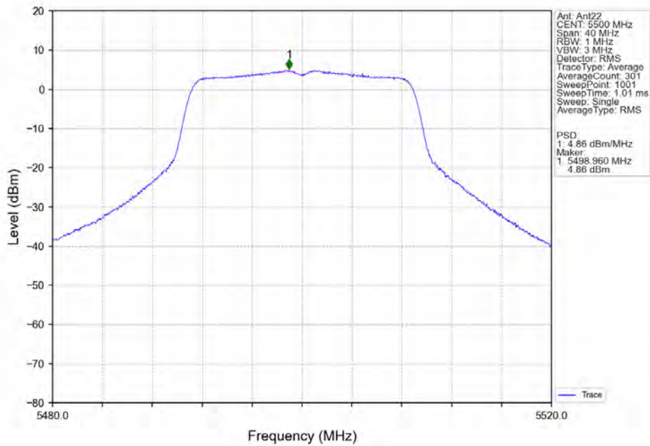
802.11n(HT20)_LCH_5500MHz_Ant22_NTNV
