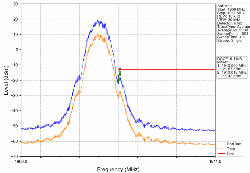
PCS1900_GSM_HCH_1909.8MHz_GSM_NTNV
