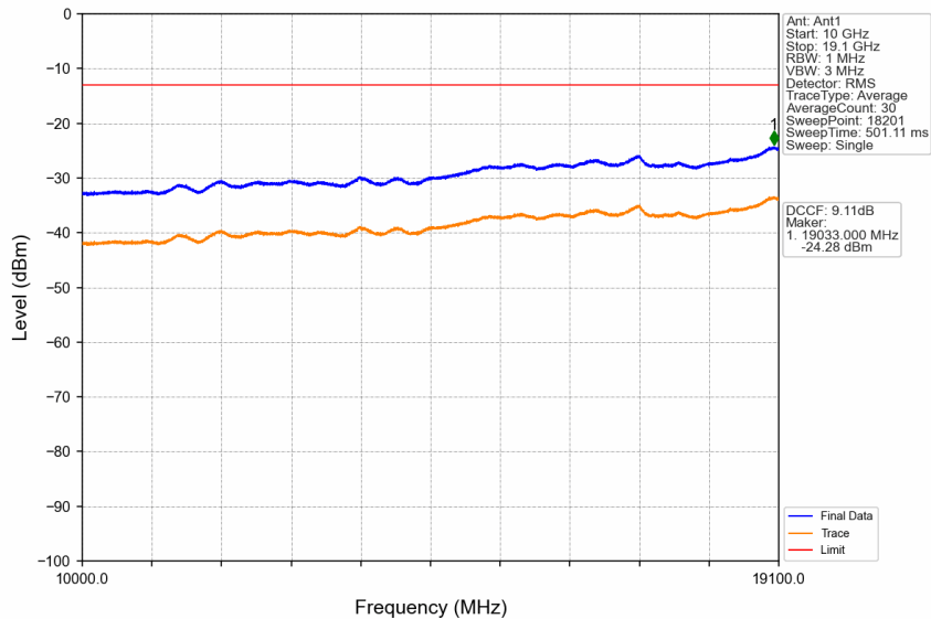
PCS1900_GSM_MCH_1880MHz_GSM_NTNV
