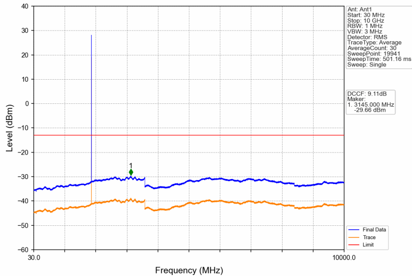
PCS1900_GSM_MCH_1880MHz_GSM_NTNV
