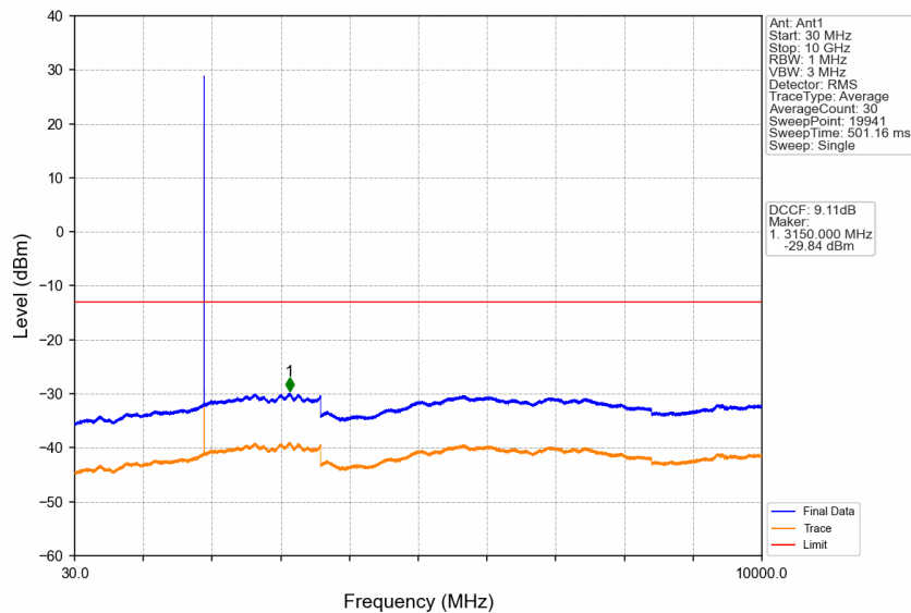
PCS1900_GSM_HCH_1909.8MHz_GSM_NTNV
