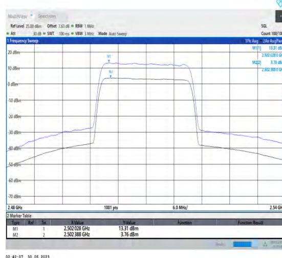
1-N7-PC3-15-20-L-2-CP-256QAM-Outer_Full-106@ 0-Ant1-9.55-100%-0.00-9.55-PASS-≤13
