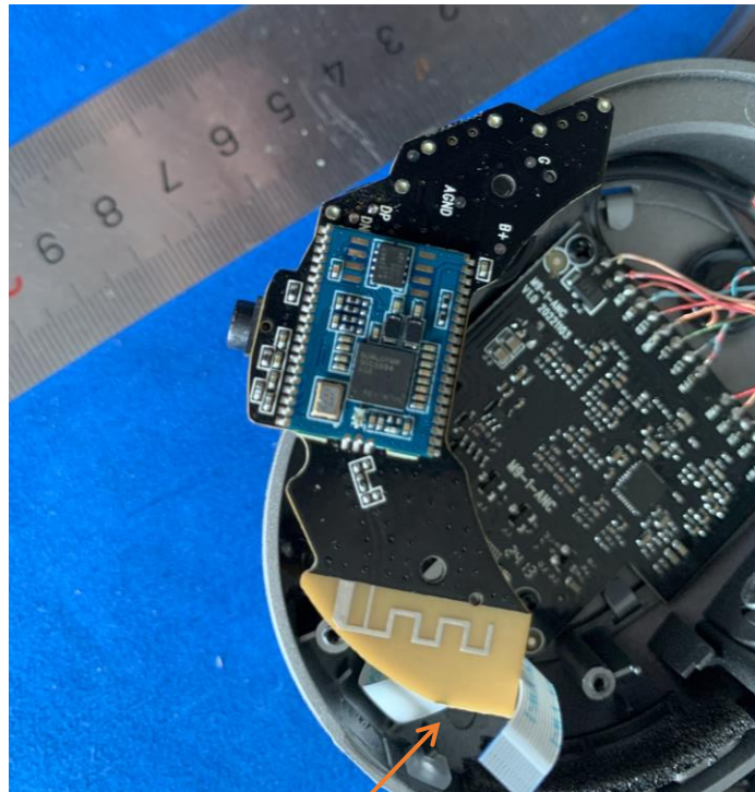
Antenna
