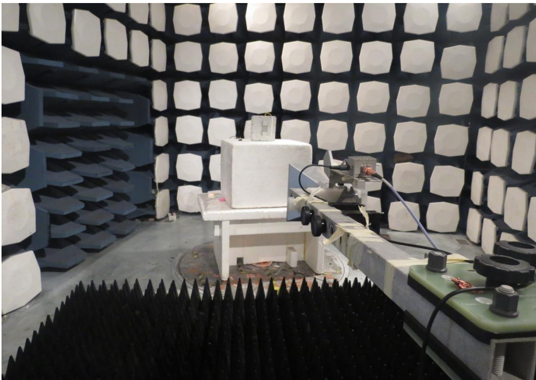
1GHz-18GHz
