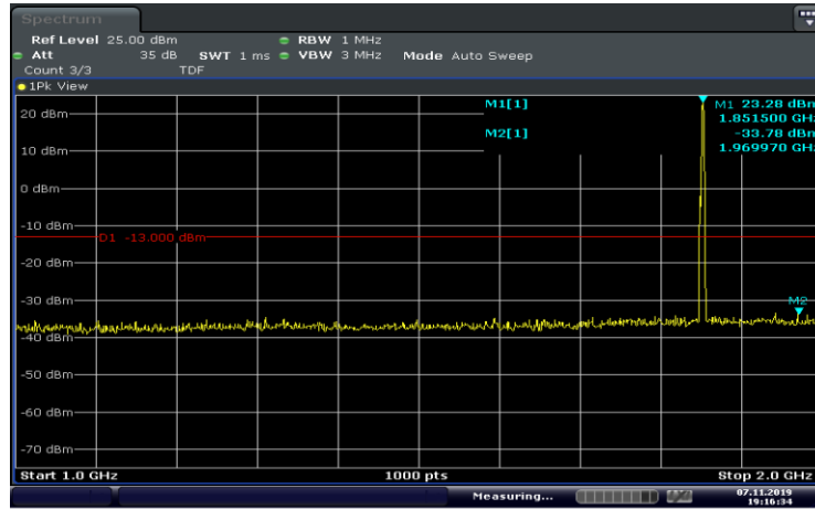
Band2-1.4MHz-QPSK-18607-6RB#0-Range2:1000~2000MHz
