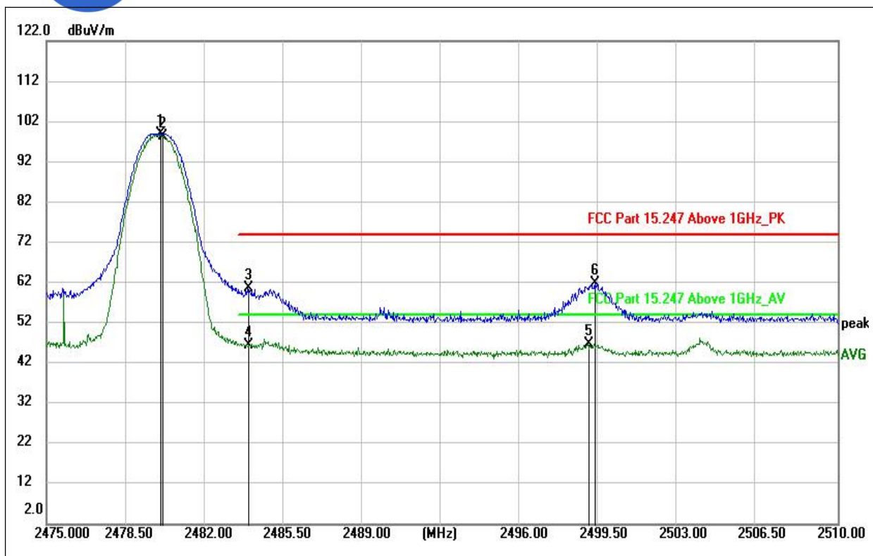
(LE 1M PHY_2480MHz, Antenna Horizontal)
