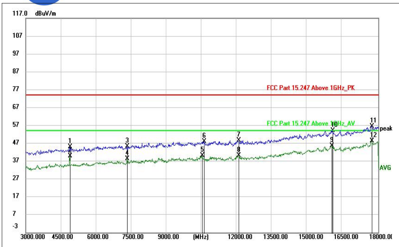
(LE 1M PHY_2442MHz, Antenna Horizontal, 3GHz to 18GHz)
