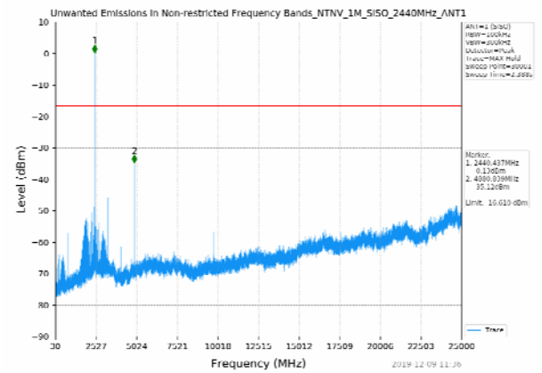
30MHz-25GHz CH19
