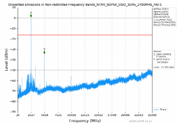
30MHz-25GHz CH78
