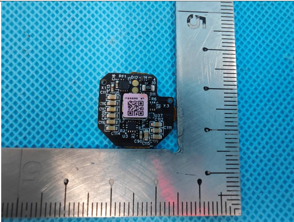
EUT Photo(6) - D2&D4
