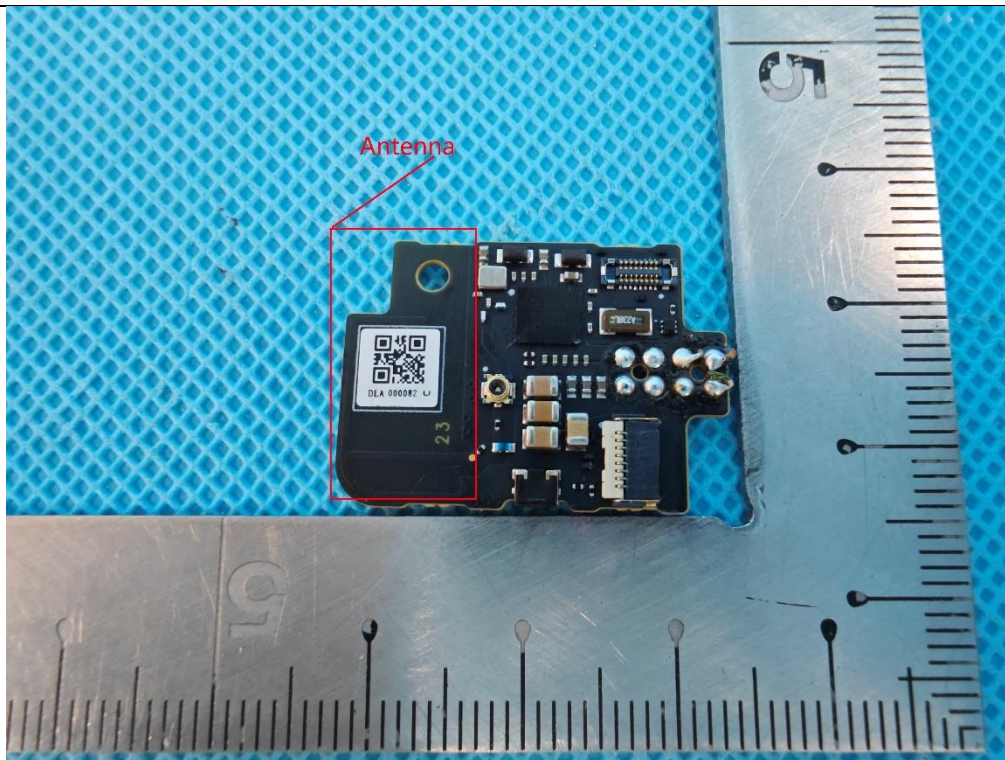
EUT Photo(8) - D2&D4 NFC Antenna
