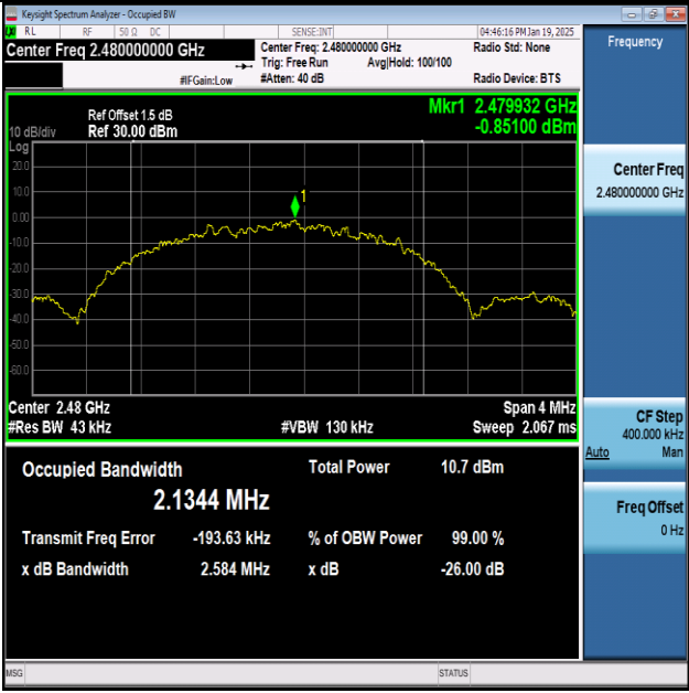
BLE_2M-Ant1-2480
